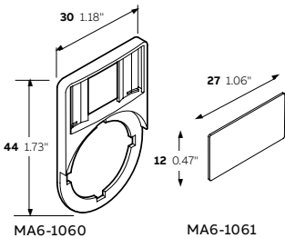
尺寸 (mm, 英寸)
