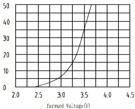
FORWARD CURRENT VS FORWARD VOLTAGE 正向电流和正向电压的关系曲线图
