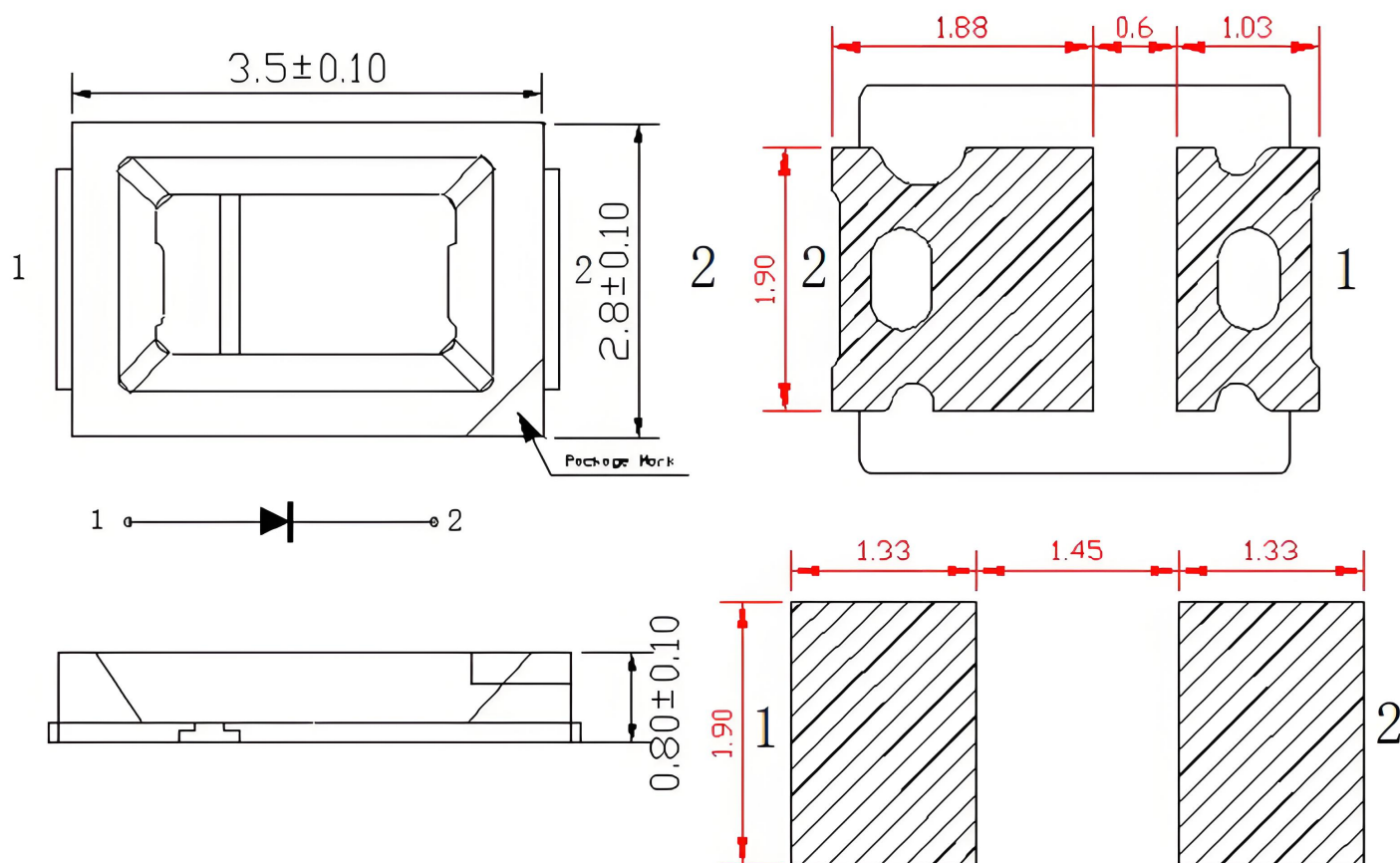
焊盘图
