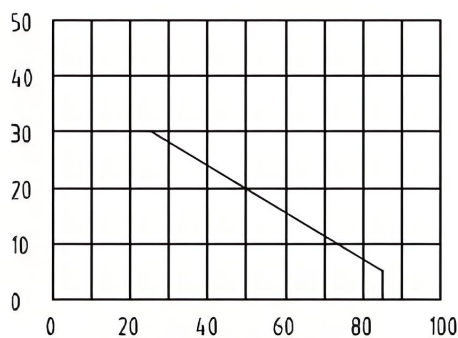
FORWARD CURRENT VS DEBATING CURVE 正向电流随温度变化曲线图
