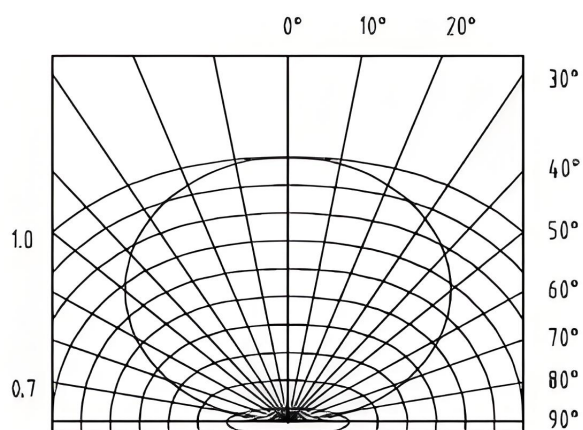
SPATIAL DISTRIBUTION 发光角度图
