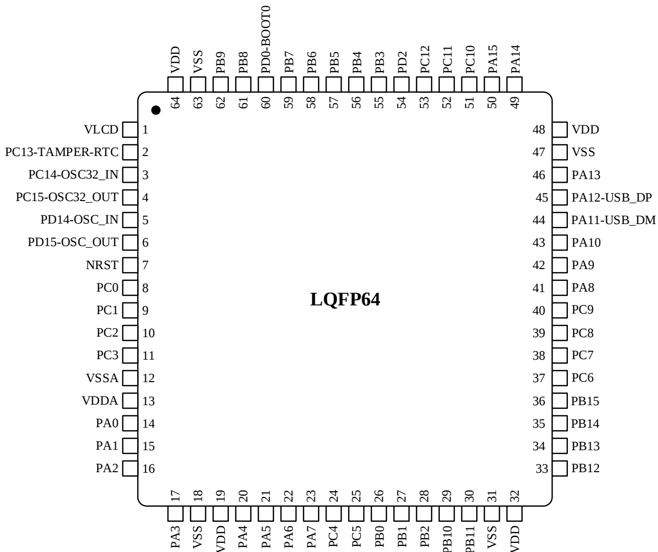
图 3-6 N32L402/N32L406(10mm x 10mm)系列 LQFP64 引脚分布
