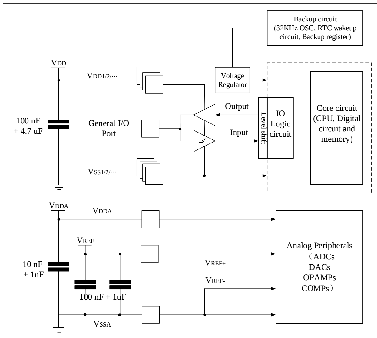
图 4-3 供电方案
