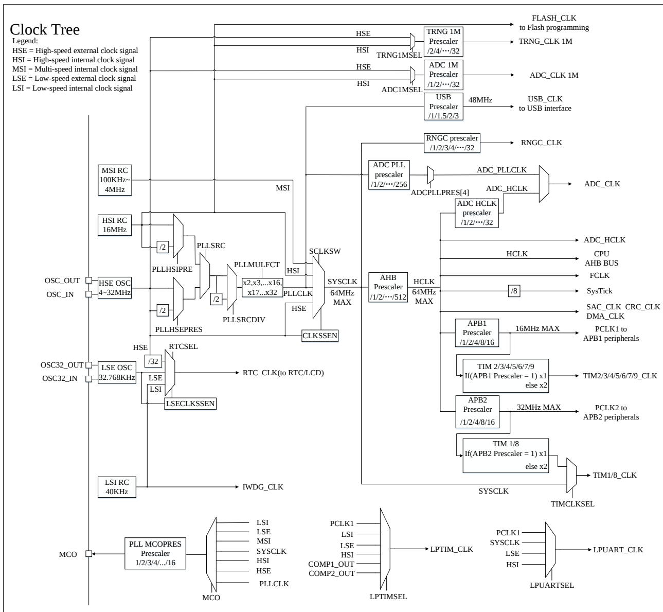
图 2-2 时钟树
