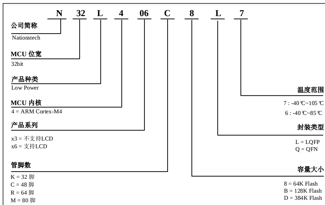
图 1-2 N32L40x 系列订货代码信息图示
