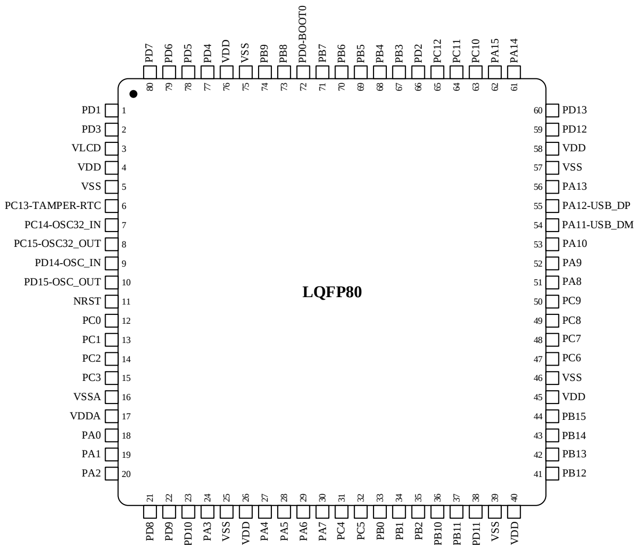
图 3-7 N32L406(12mm x 12mm)系列 LQFP80 引脚分布
