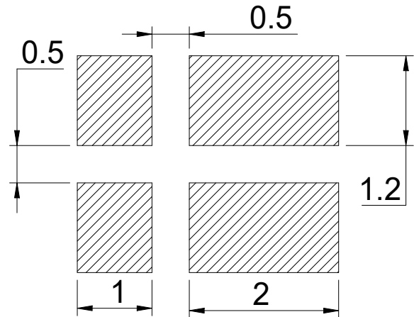
焊盘建议图
