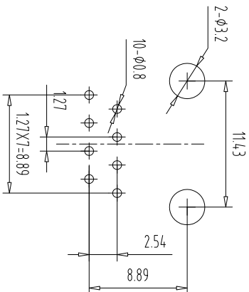
P. C. B参考图
