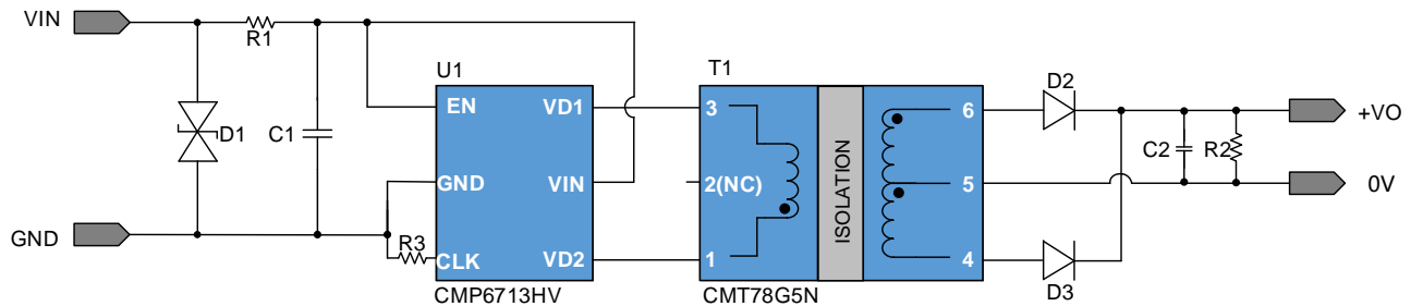
图 3.1 CMP6713HV 12V 输入, 5V 输出 2W 方案原理图
