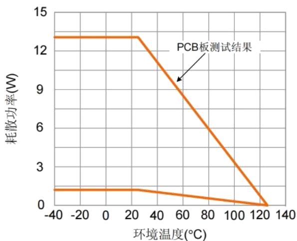
耗散功率 VS 环境温度 (TO-252)
