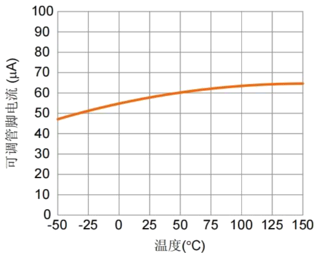
可调管脚电流
