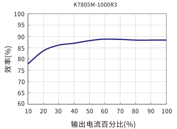
效率Vs输出负载 (标称输入)
