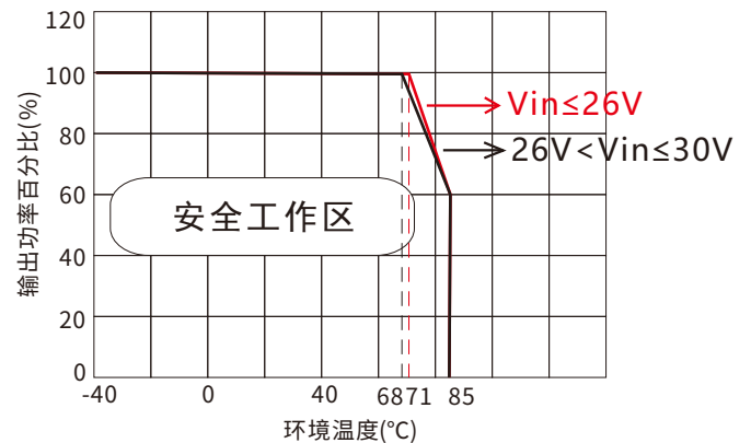
6.5V/9V/12V/15V 正输出 温度降额曲线图
