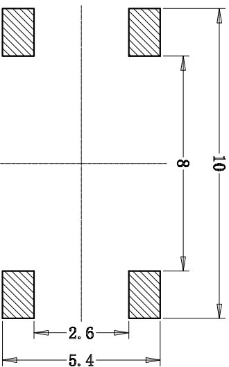
RECOMMENDED P.C.B. LAYOUT 安装尺寸图
