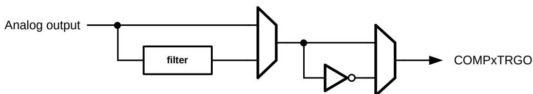
图 16-4 比较器触发输出信号产生
