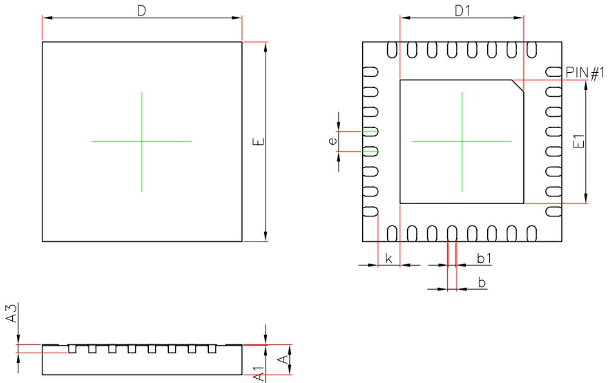
图 2-4 QFN32 封装尺寸图
