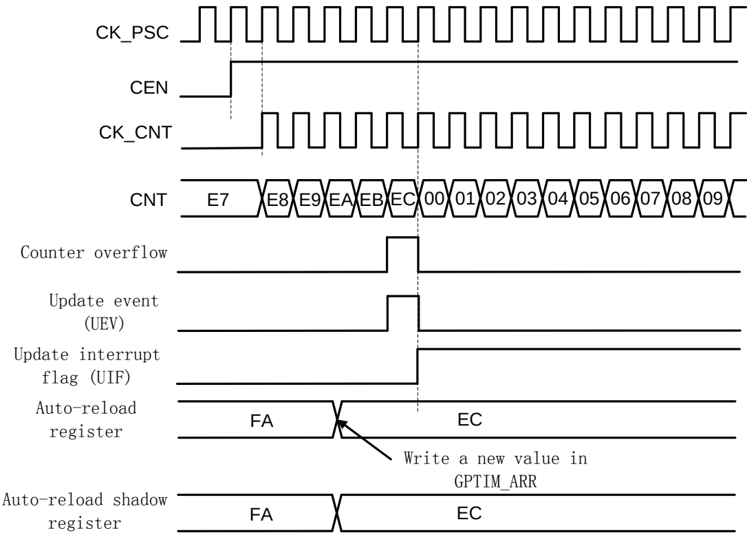
图 28-6 ARPE=0（GPTIM_ARR 没有预装载）时的更新事件
