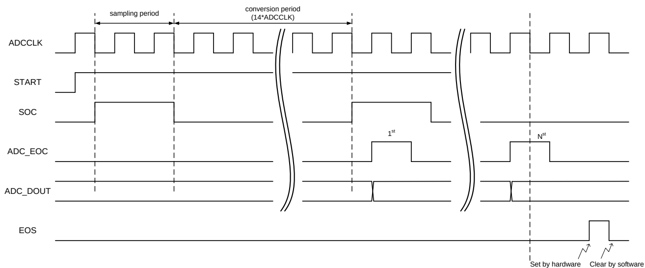
图 32-4 ADC 采样序列时序
