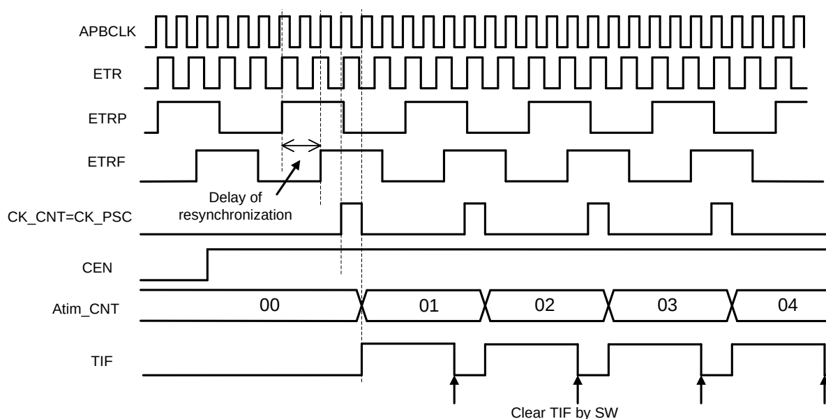
图27-23外部时钟模式2下的时序2
