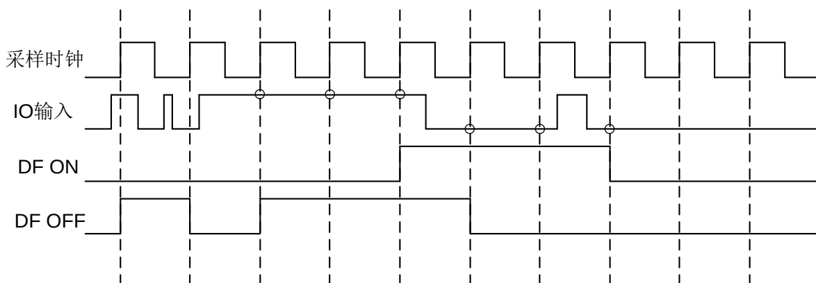
图 33-4 引脚输入数字滤波
