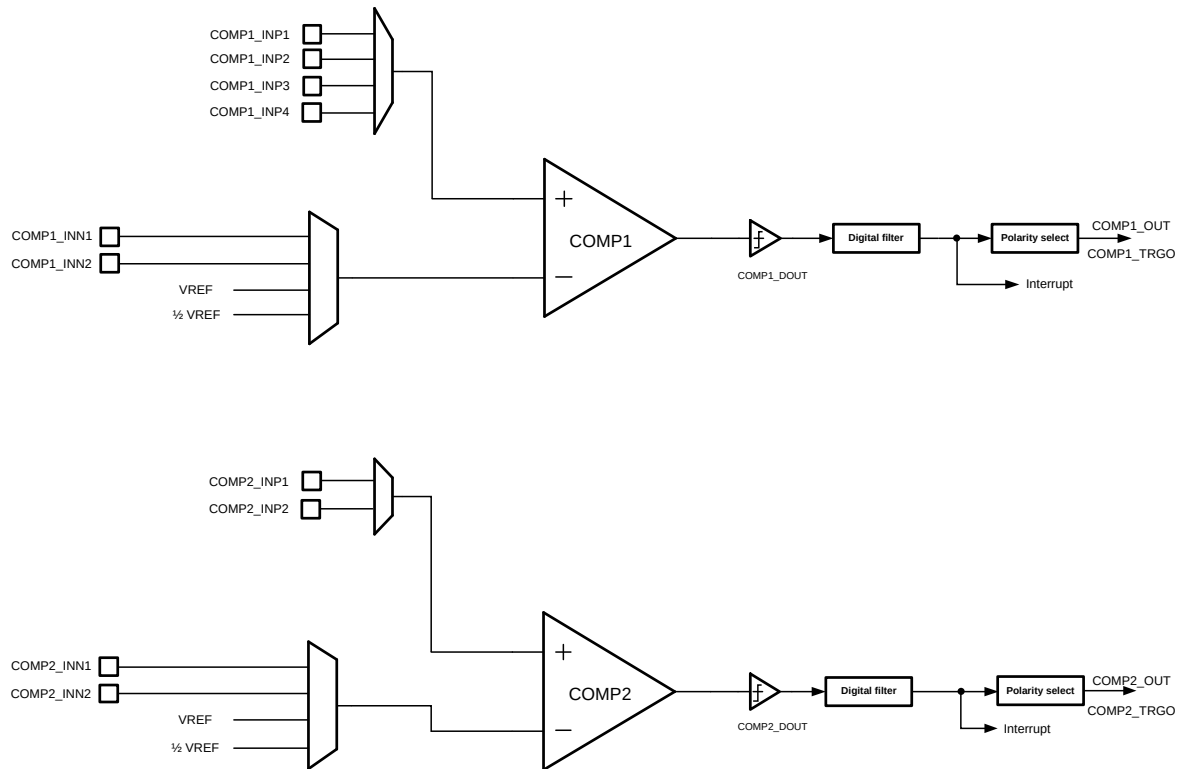
图 16-1 比较器电路框图
