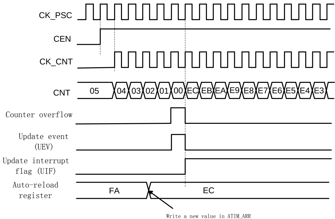
图 27-10 向下计数，内部时钟 2 分频
