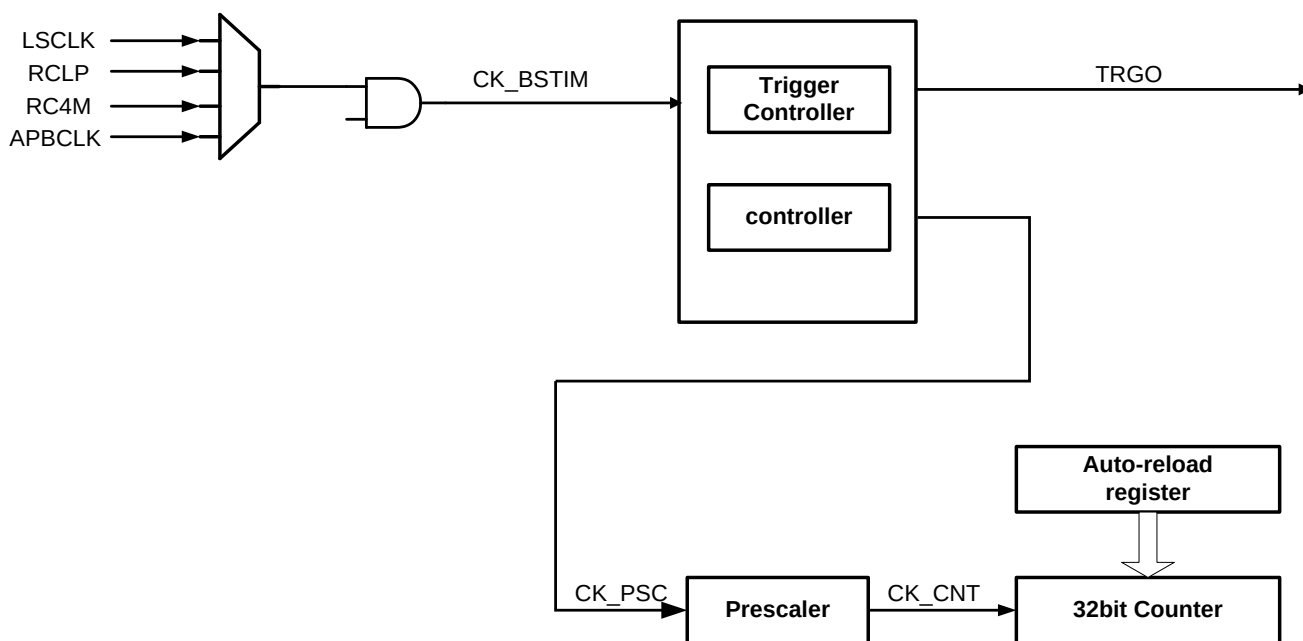
图29-1BSTIM32结构框图
