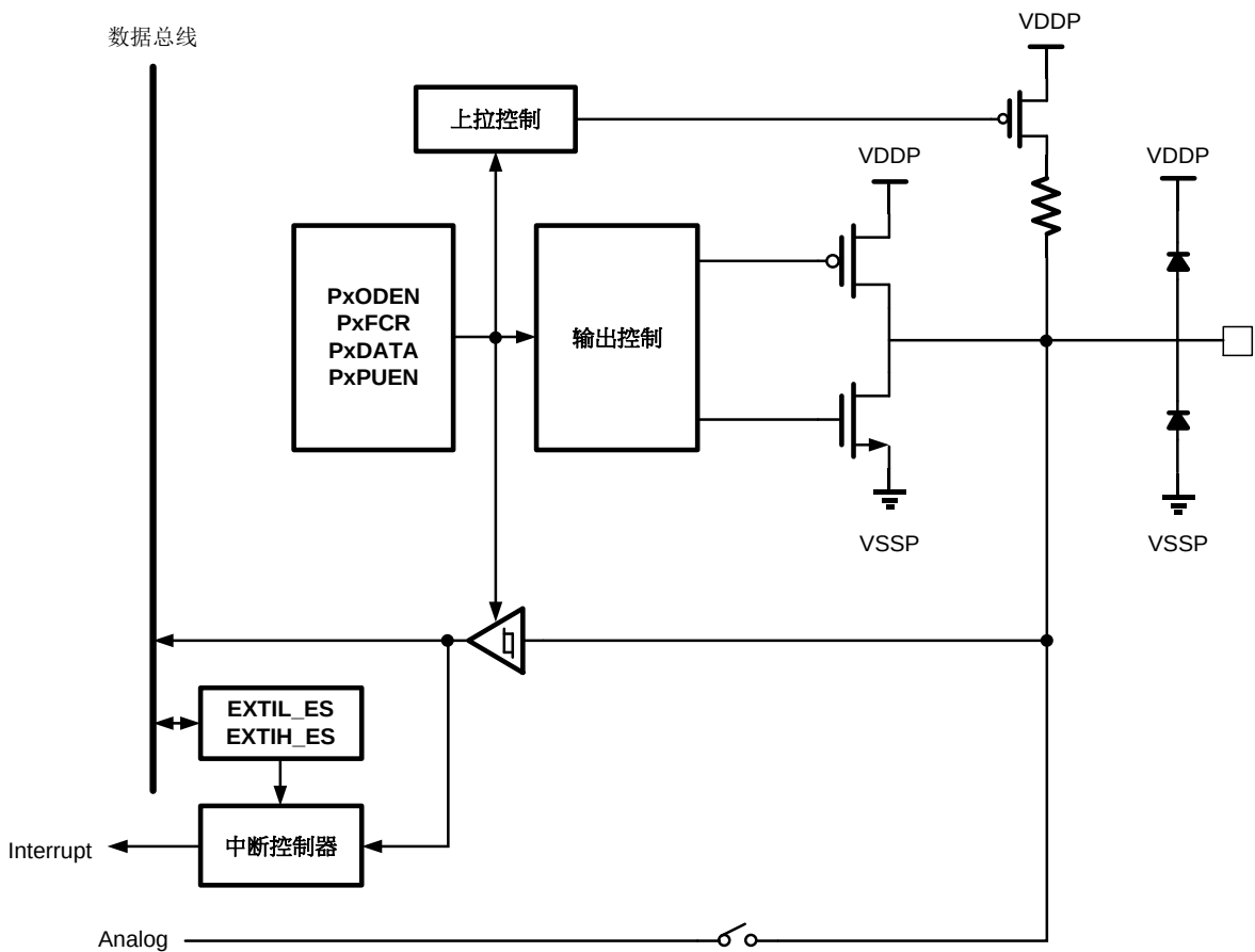
图 33-1 普通 GPIO 结构框图
