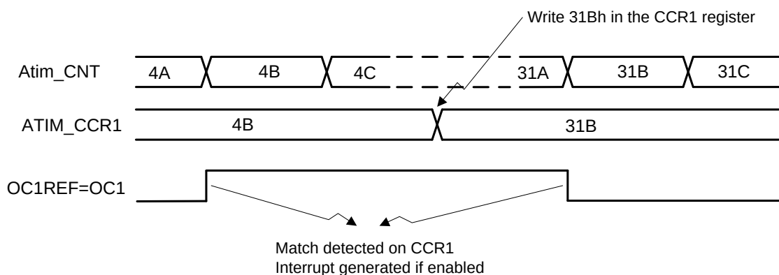
图27-29输出比较模式，翻转OC1
