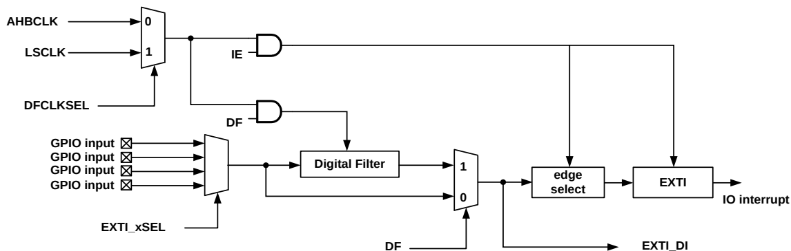
图 33-5 EXTI 信号输入示意图
