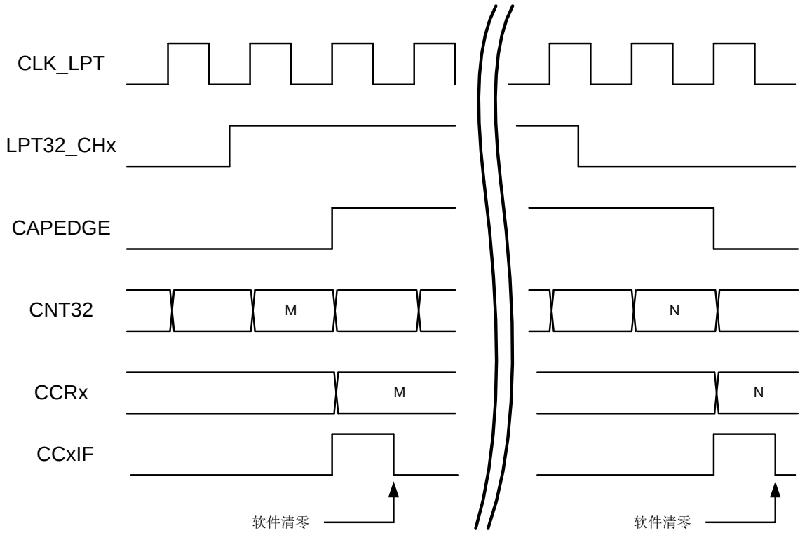
图 30-6PWM 输出
