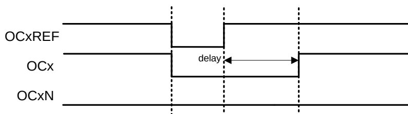
图27-33死区波形延迟大于负脉冲
