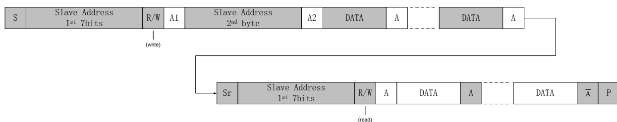
图 18-19 I 2 C 软件发送数据流图
