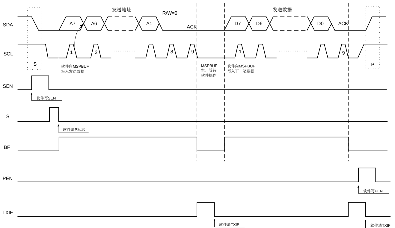
图 19-9I2C 主机对 7 位地址从机发送数据流程图
