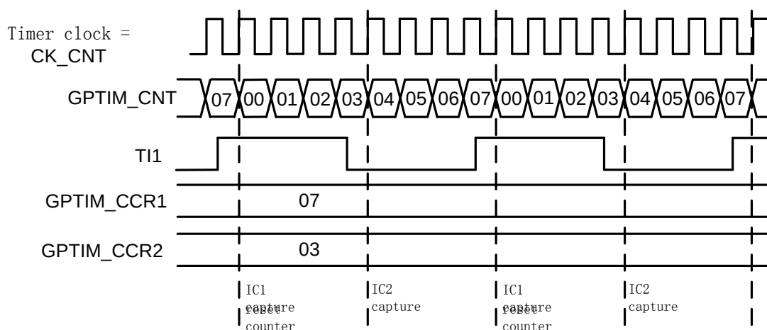
图28-26 PWM输入捕获模式时序
