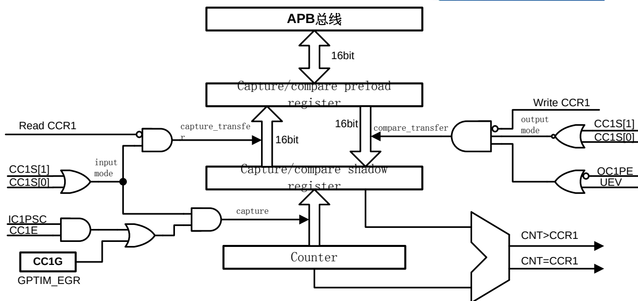
图28-24捕获/比较通道1的主电路
