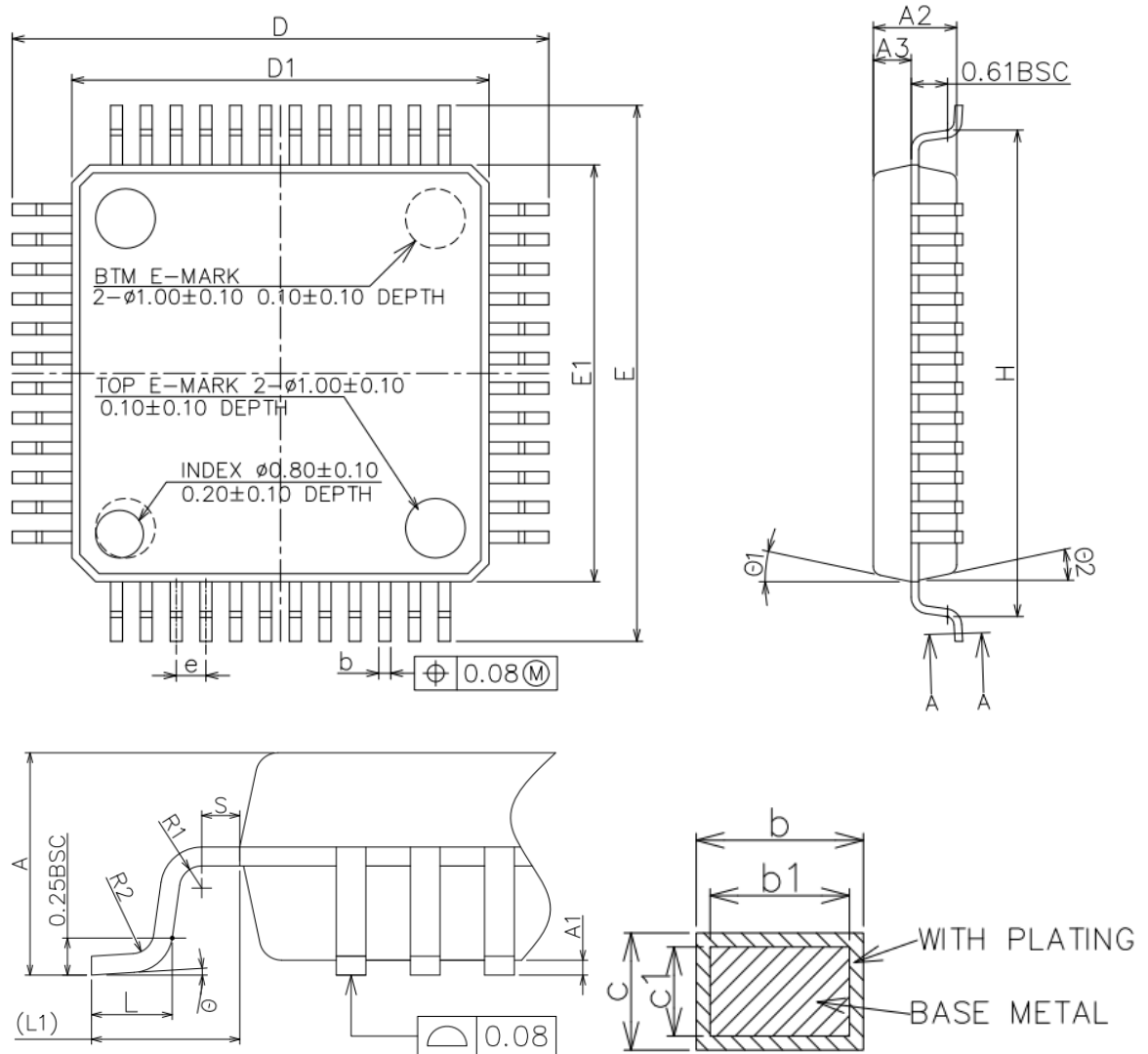
图 2-3LQFP48 封装尺寸图
