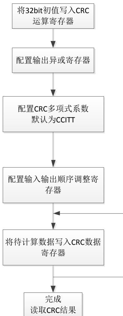
图 26-1CRC 运算流程图
