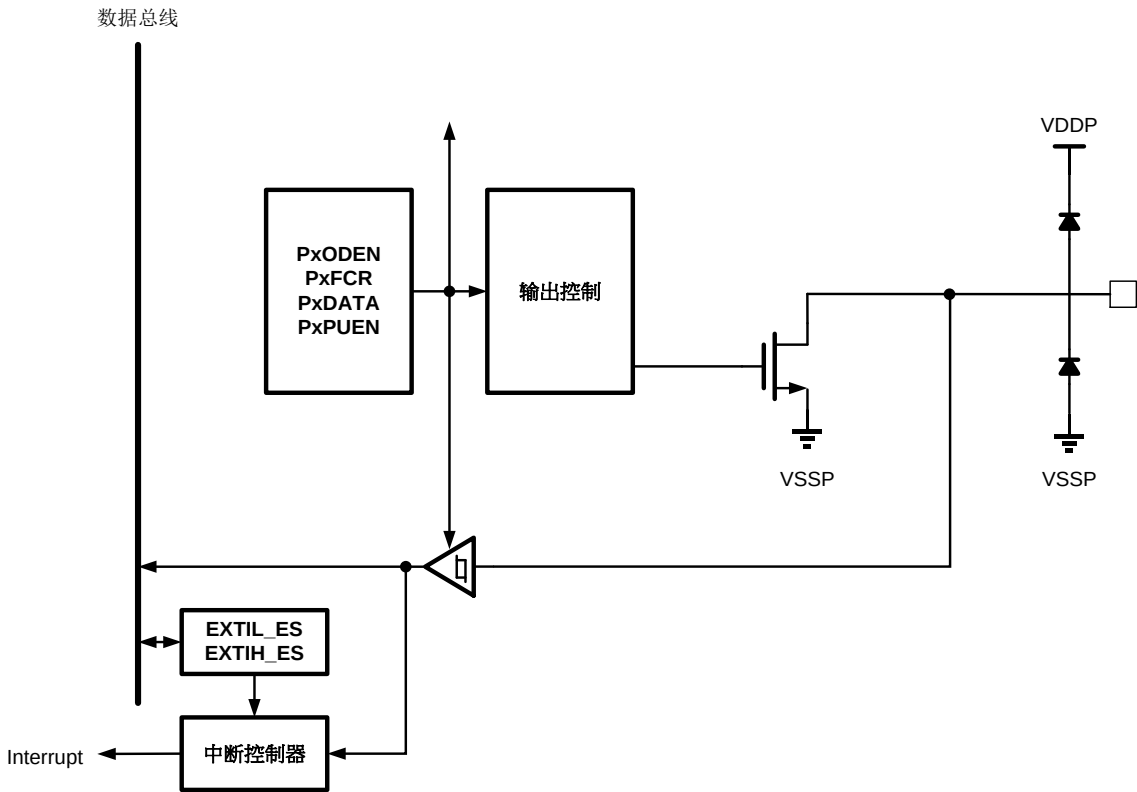
图 33-2PA11 PA12 结构框图
