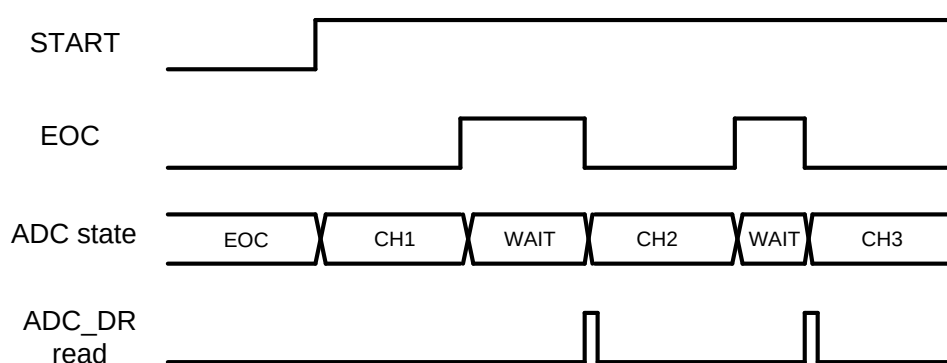
图 32-9 ADC 自动等待
