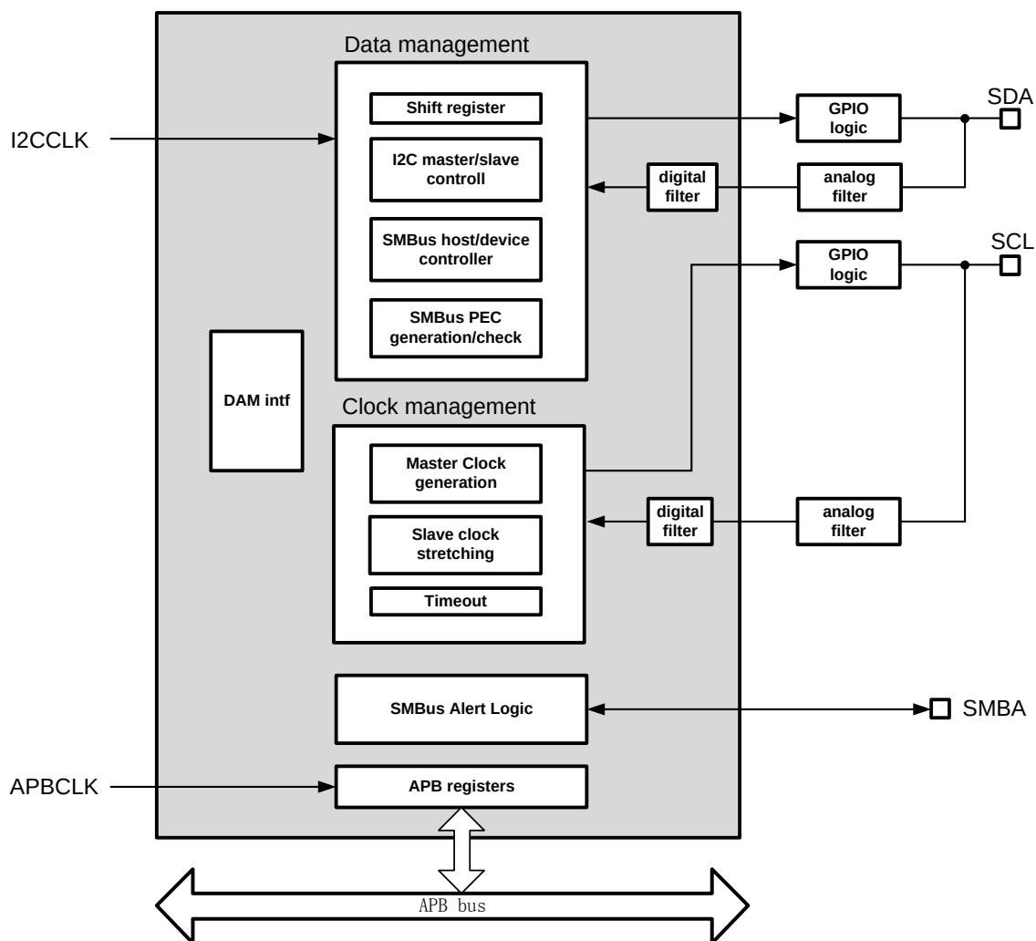
图 18-1 I 2 C-SMB 模块框图
