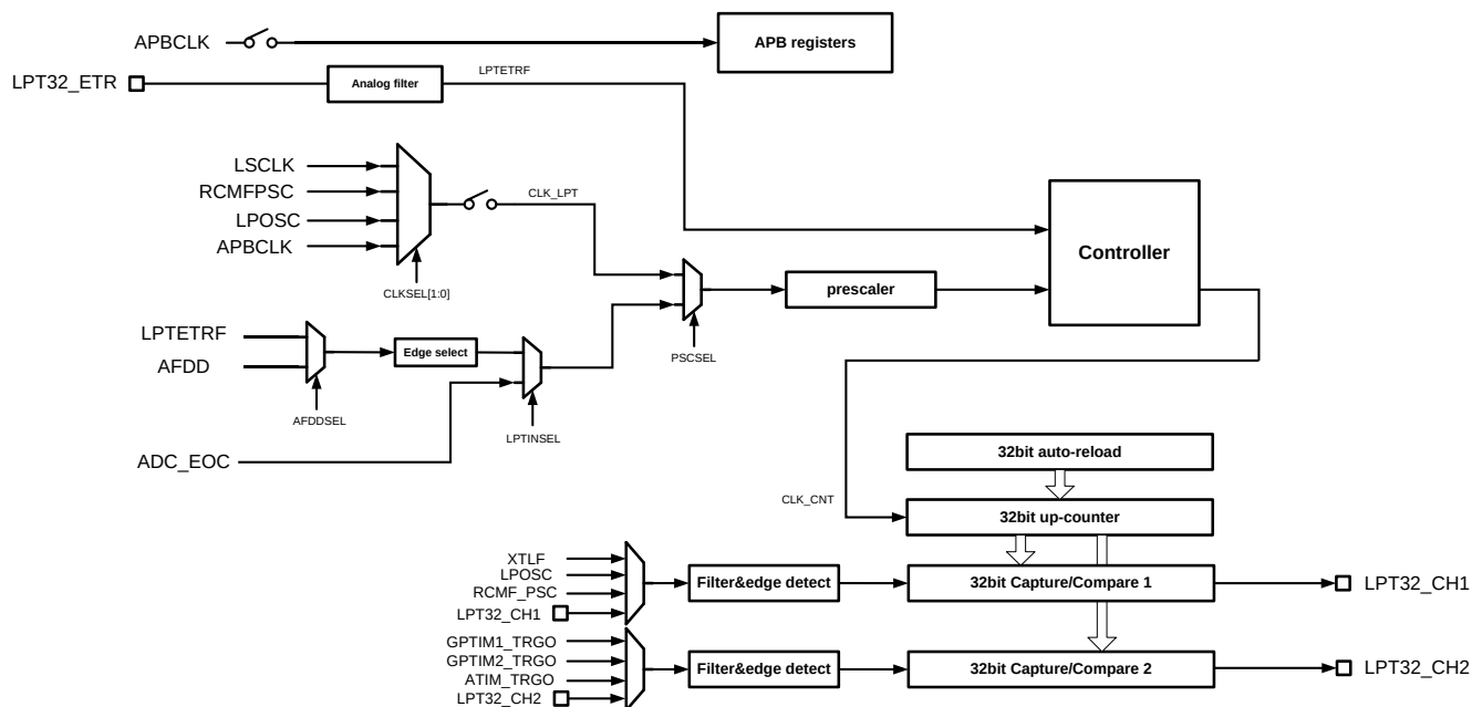
图 30-1LPTIM32 结构框图
