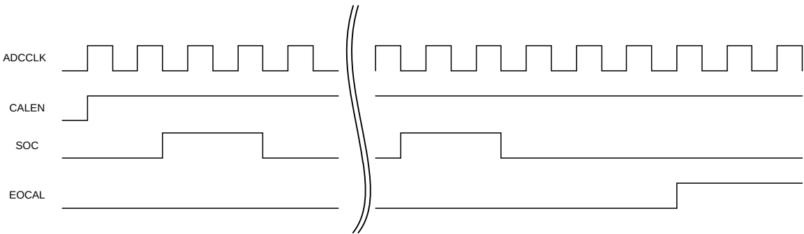
图 32-2 ADC 校准时序
