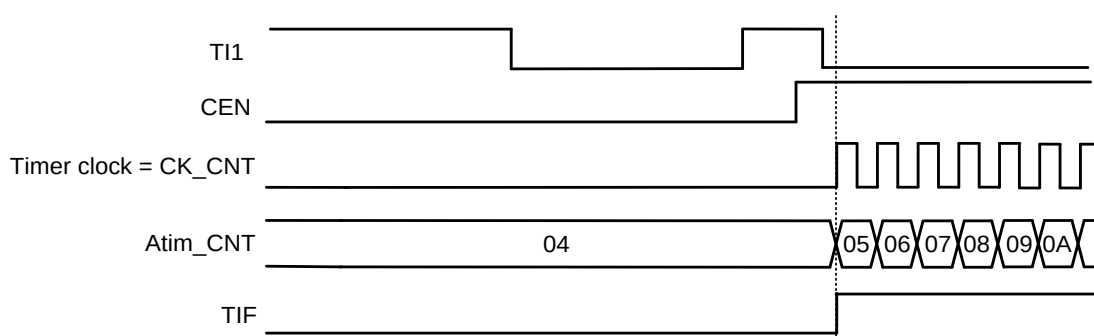
图28-35 触发器模式下的时序
