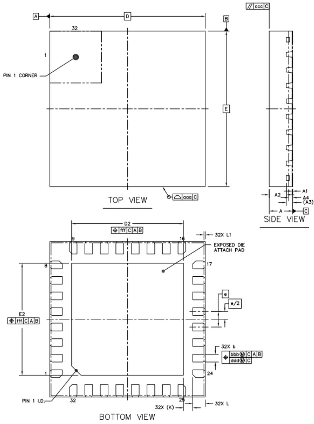
图 2-5 QFN32 (wettable flank) 封装尺寸图
