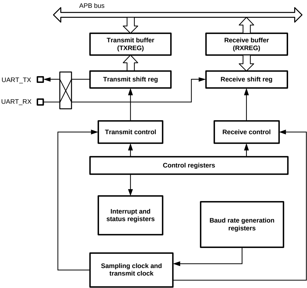
图 20-1 UART 结构框图
