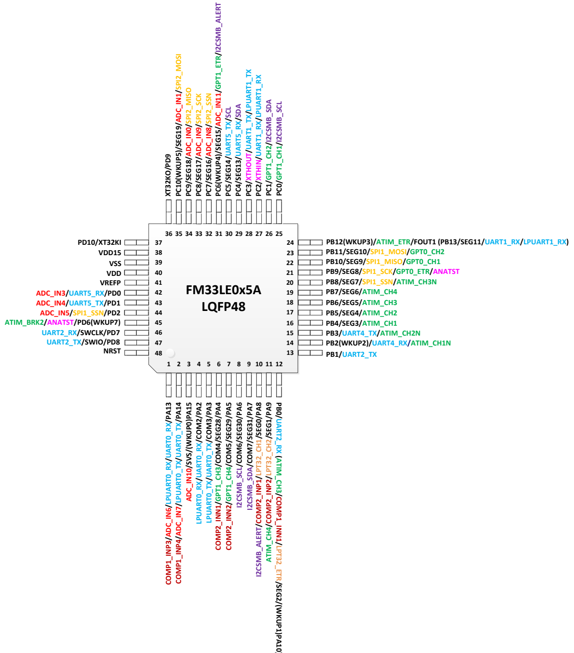
图 2-1FM33LE0x5A LQFP48 封装图
