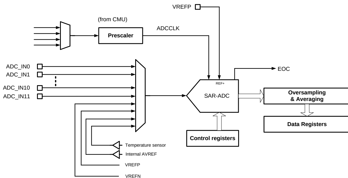
图 32-1 ADC 模块框图
