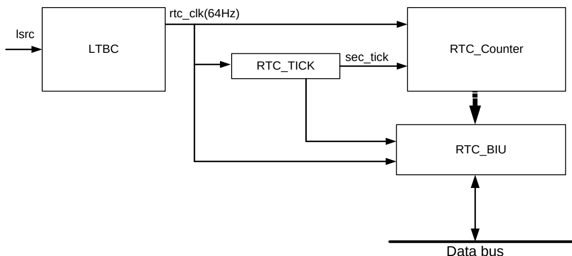
图 31-1 RTC 结构框图
