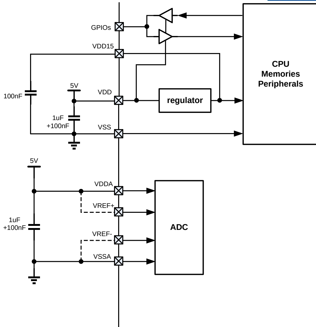
图 3-1FM33LE0A 供电方案
