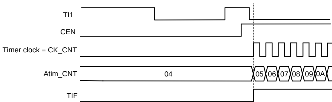
图27-42触发器模式下的时序
