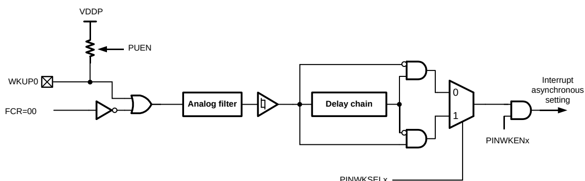
图 33-3WKUPx 功能结构框图
