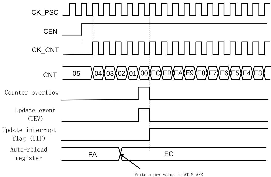
图 27-11 向下计数，不使用重复计数时的更新事件
