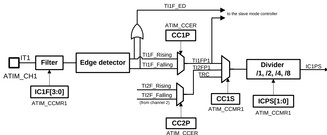
图27-24捕捉/比较通道(通道1输入部分)
