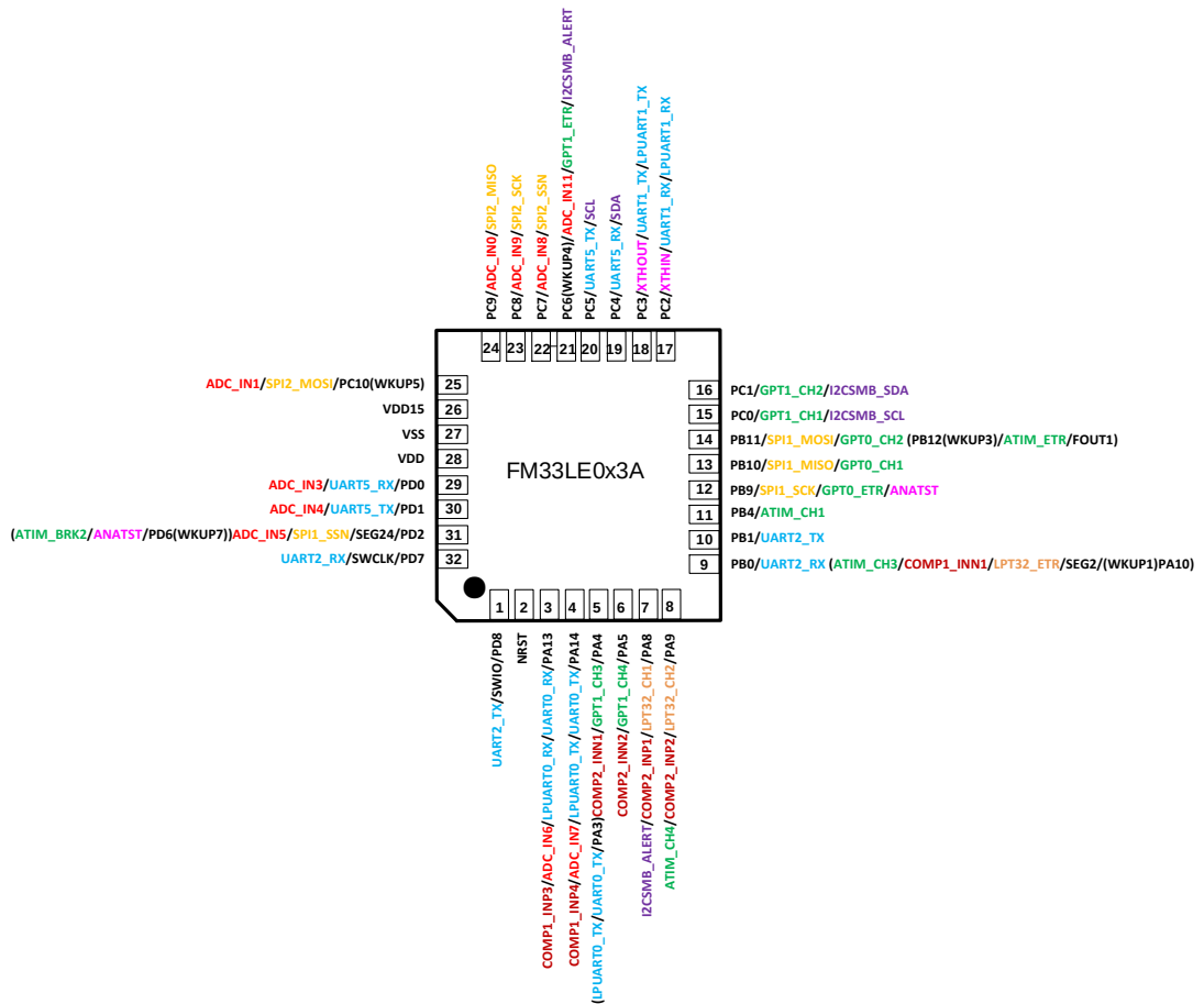
图 2-2FM33LE0x3A QFN32 封装图
