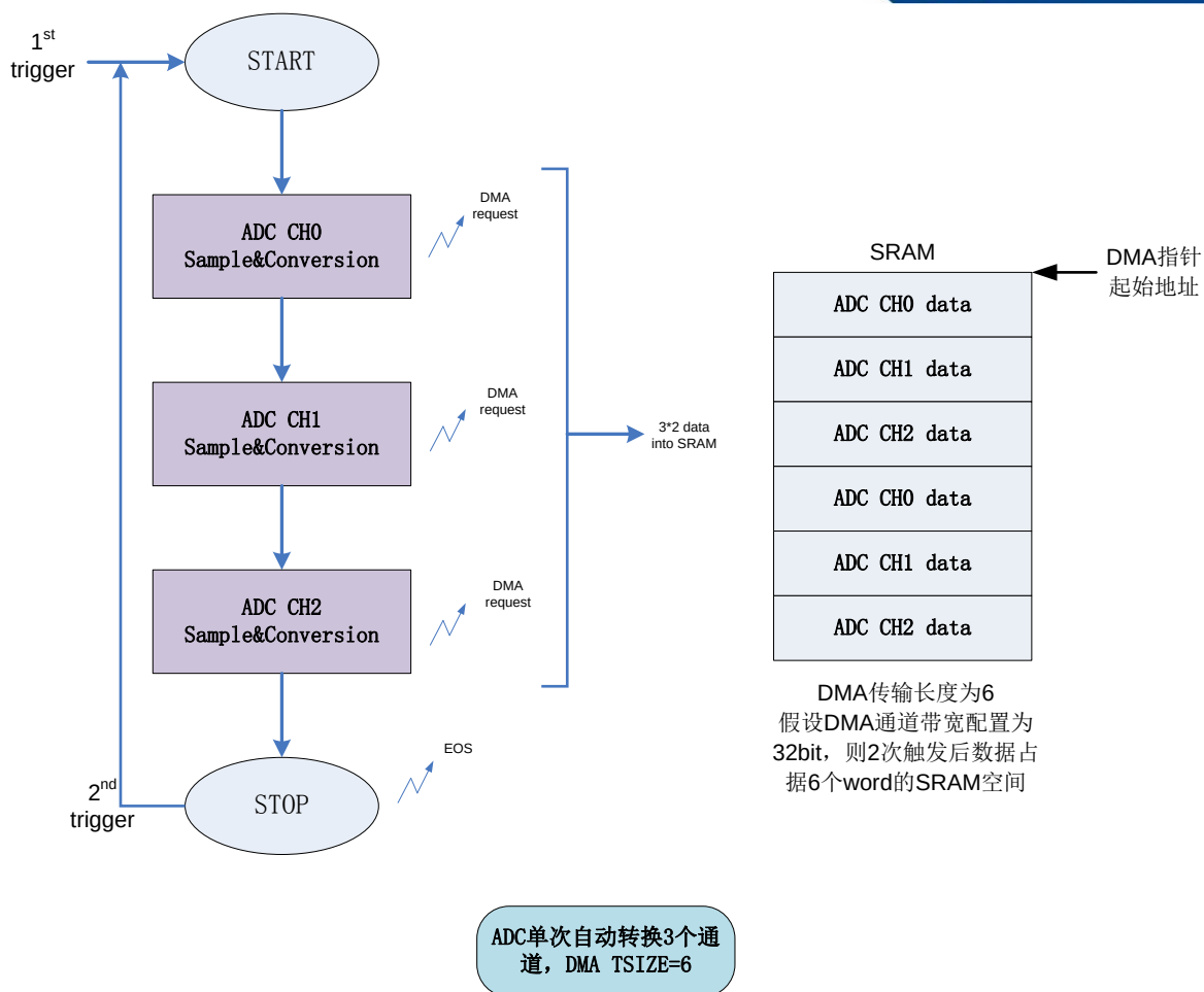
图 32-10 ADC 单次全自动触发+DMA 案例 1
