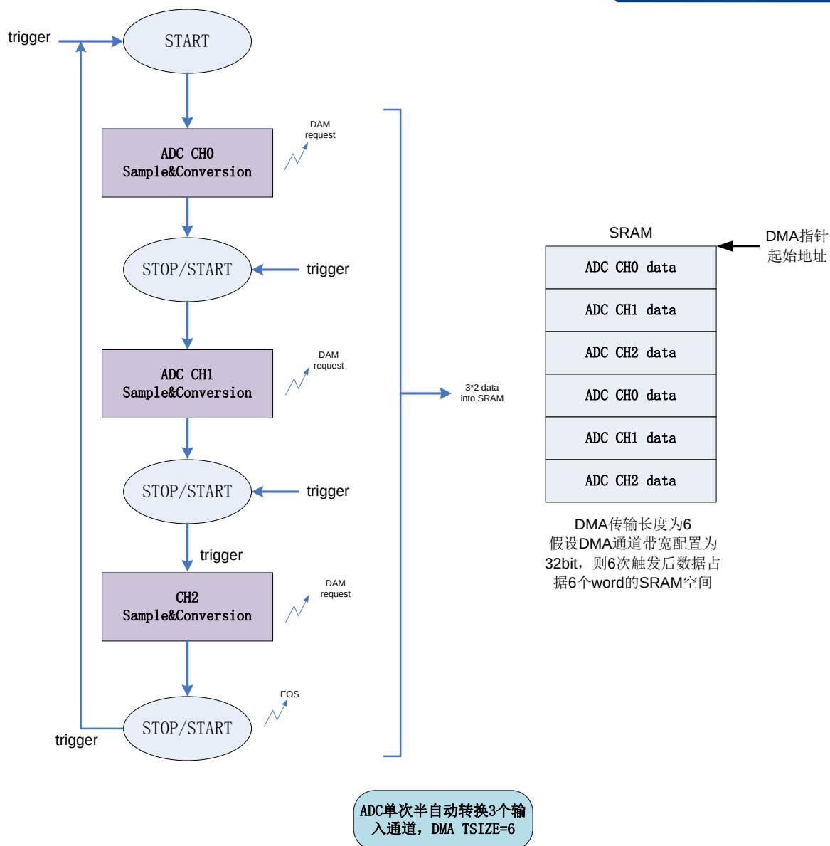
图 32-12 ADC 单次半自动触发+DMA
