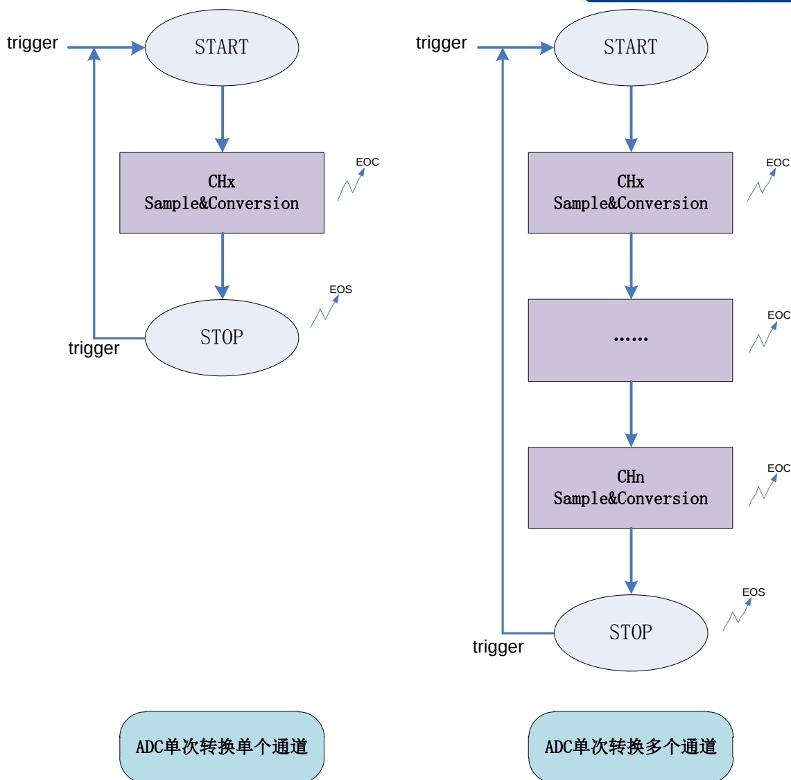
图 32-6 ADC 单次转换全自动触发模式
