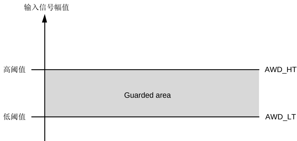
图 32-13 ADC 模拟看门狗阈值示意图
