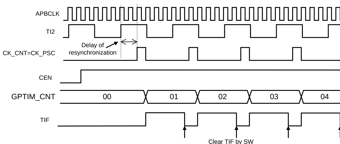
图 28-19 外部时钟模式 1 下的时序
