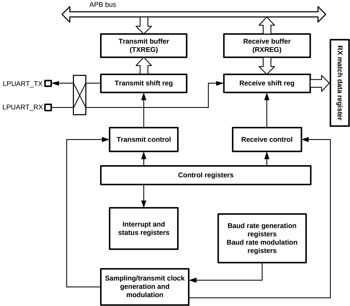
图 22-1LPUART 结构框图
