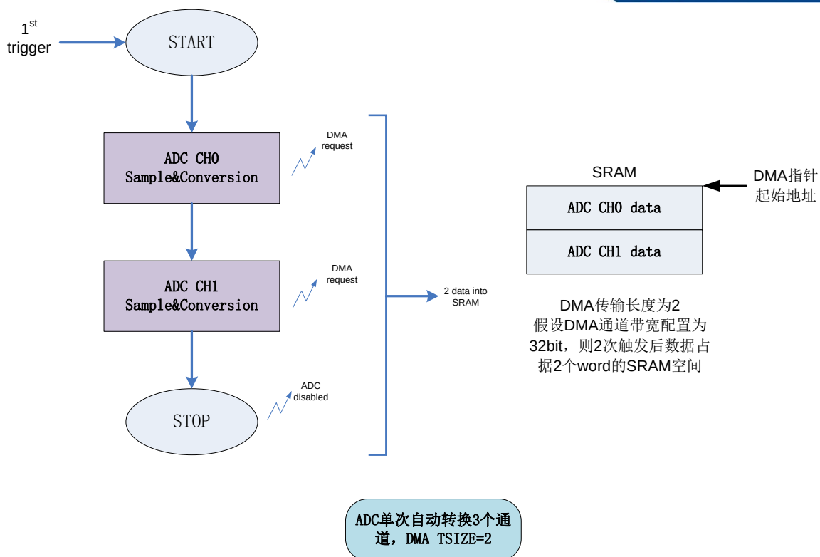
图 32-11 ADC 单次全自动触发+DMA 案例 2
