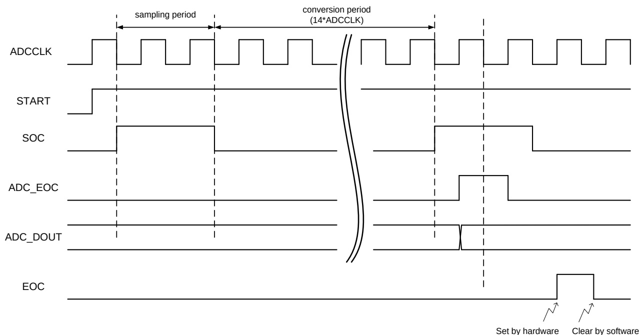
图 32-3 ADC 采样转换时序
