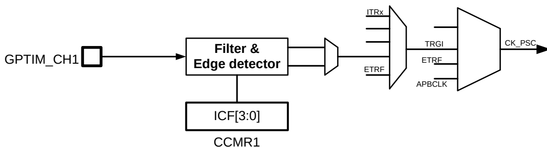
图 28-15 GPTIM 时钟源框图
