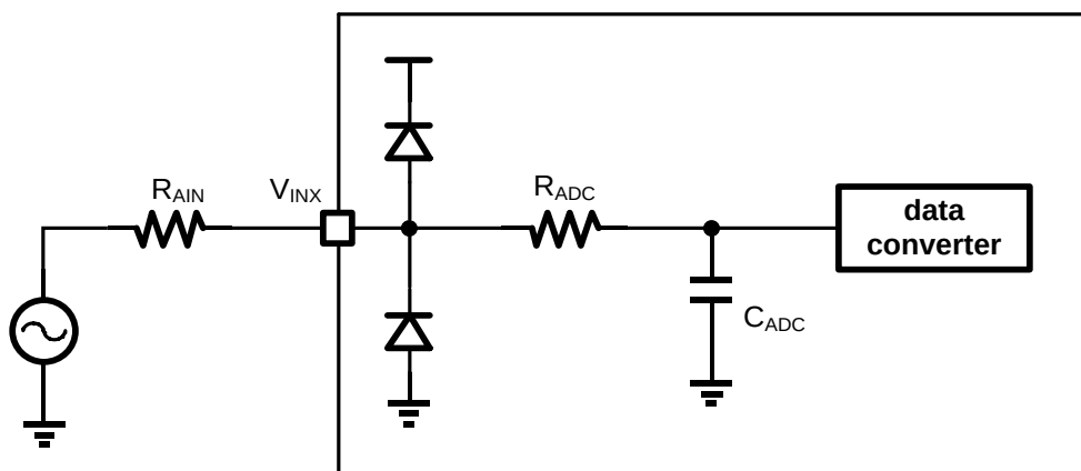
图 32-5 ADC 输入通道示意图
