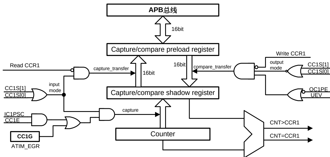
图27-25捕捉/比较通道1的主电路
