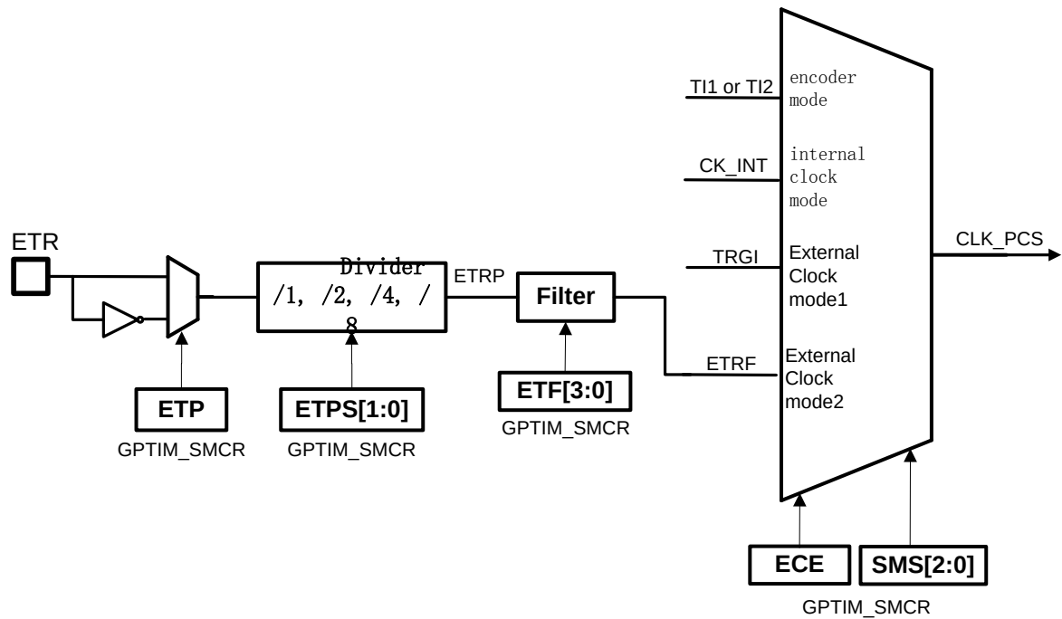
图 28-20 外部触发输入框图
