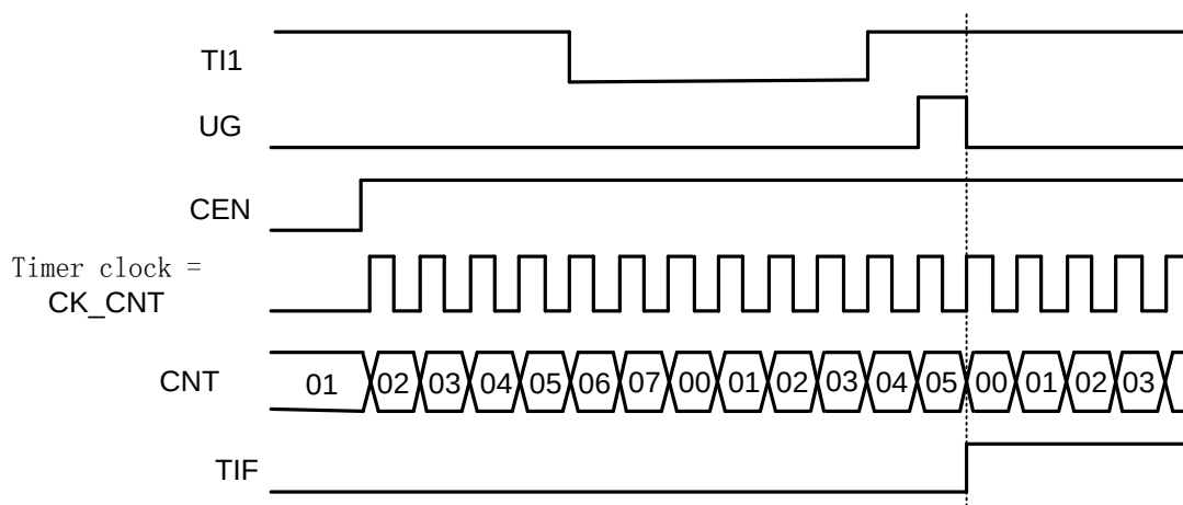
图28-33 复位模式下的时序
