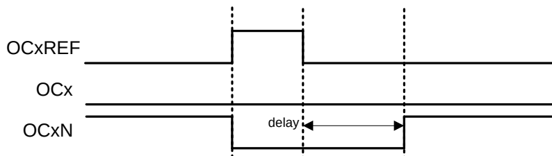
图27-34死区波形延迟大于正脉冲
