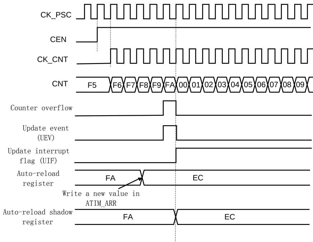
图 28-7 ARPE=1（GPTIM_ARR 预装载）时的更新事件
