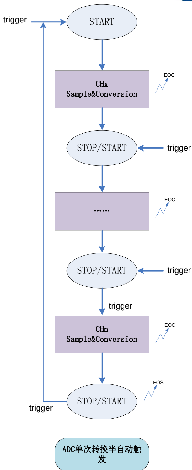
图 32-7 ADC 单次转换半自动触发模式
