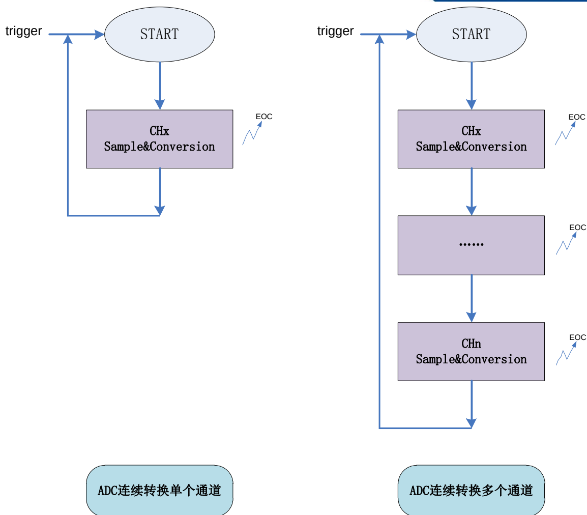
图 32-8 ADC 连续转换模式
