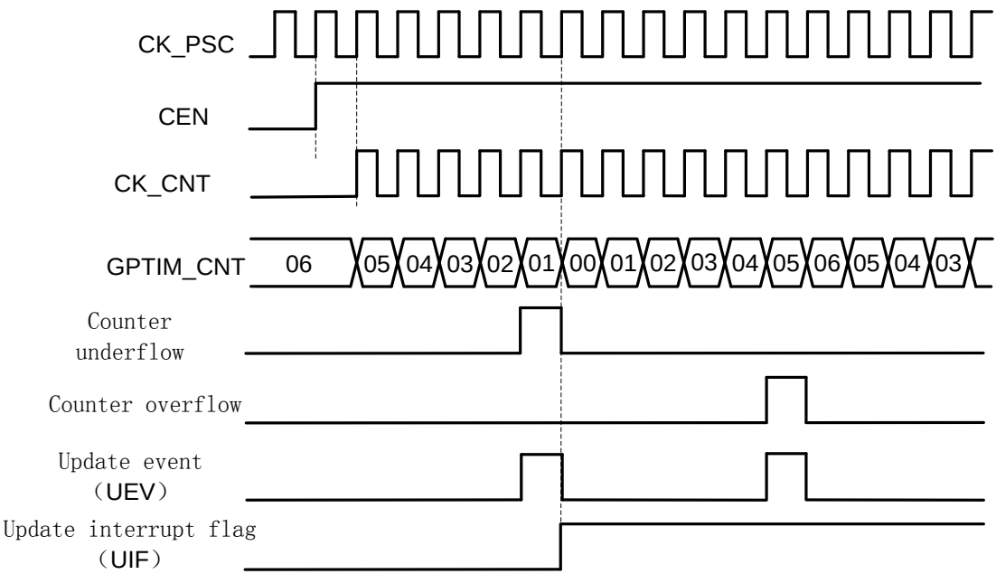
图 28-12 中心对齐计数器时序图，GPTIM_PCS=0，GPTIM_ARR=0x6
