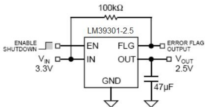
LM39301-2.5
