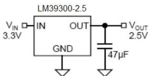
LM39300-2.5
