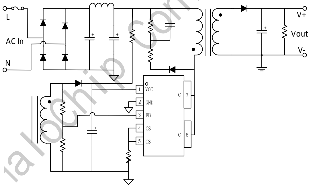
图 1 GP8691TK 典型应用图
