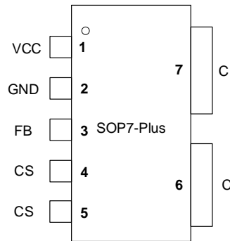
图 2 管脚封装图
