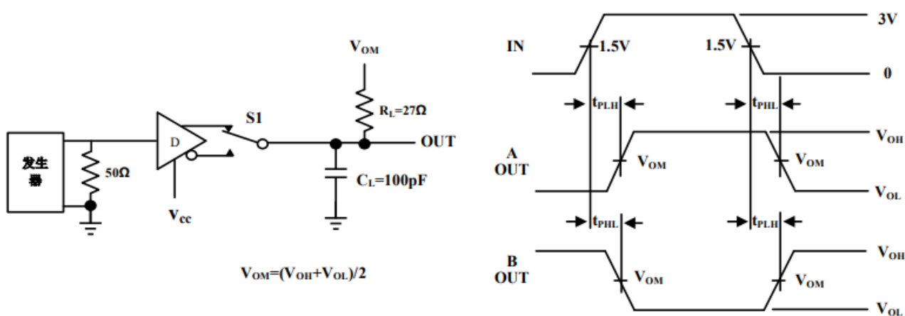
图 4 驱动器传播延迟
