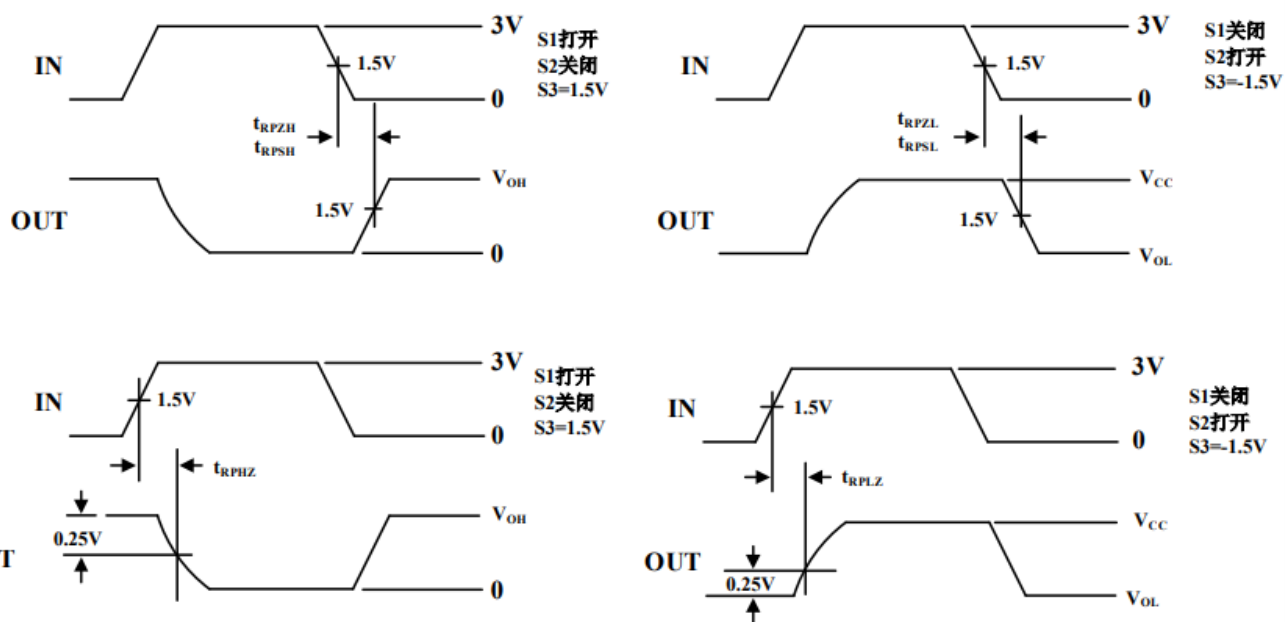
图 8 接收器使能与禁能时间
