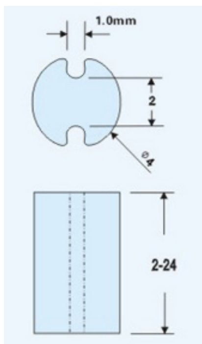
尺寸图
