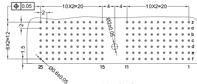
固定PCB 板尺寸 (公差±0.05)
