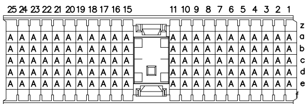
插针布局图
