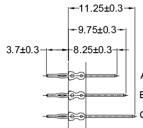
插针规格
