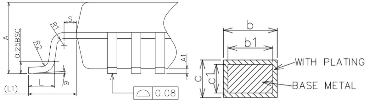
图 2-7LQFP48 封装尺寸图
