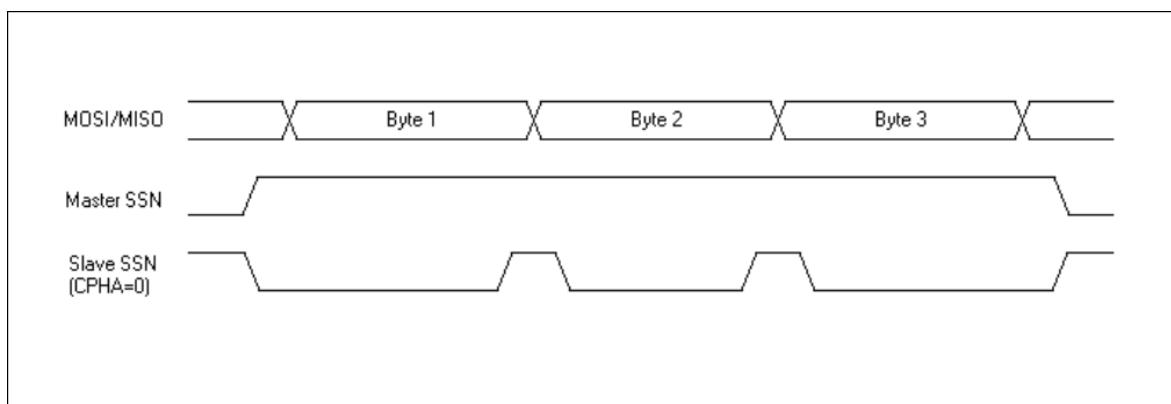
图 23-8 SPI SSN 时序图（SSNM=1，CPHA=0）
