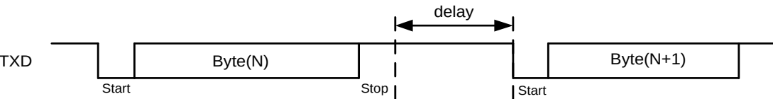
图 20-8 UART 发送延迟
