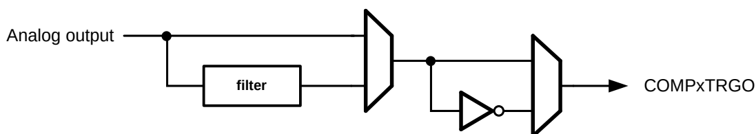
图 16-4 比较器触发输出信号产生
