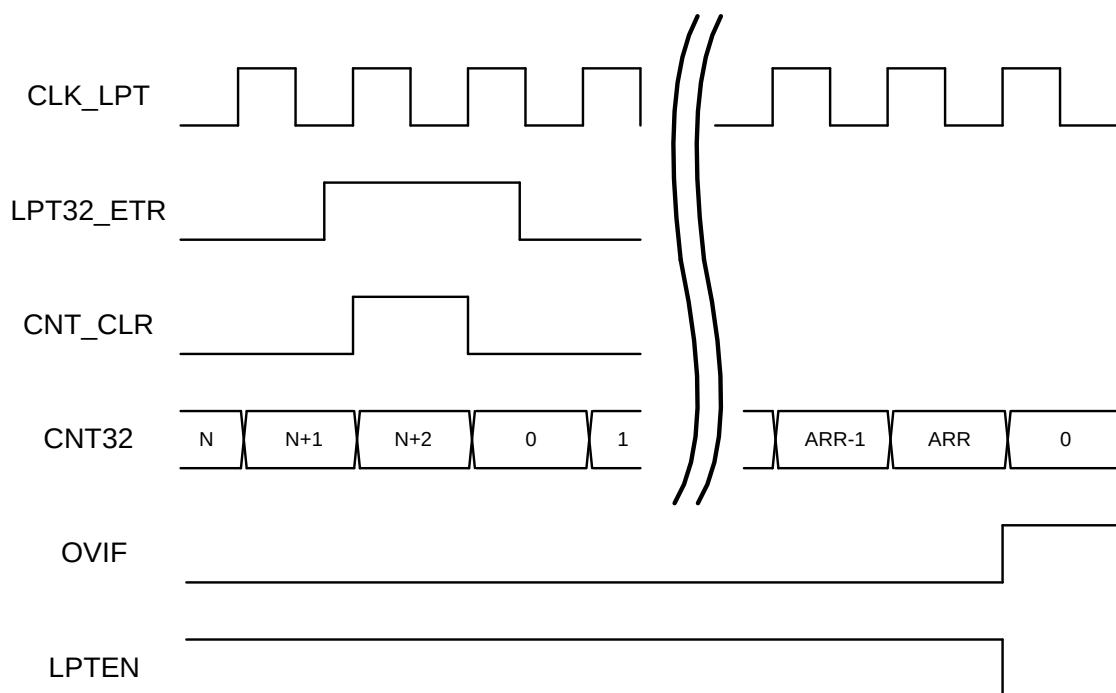
图 30-4TimeOut 模式
