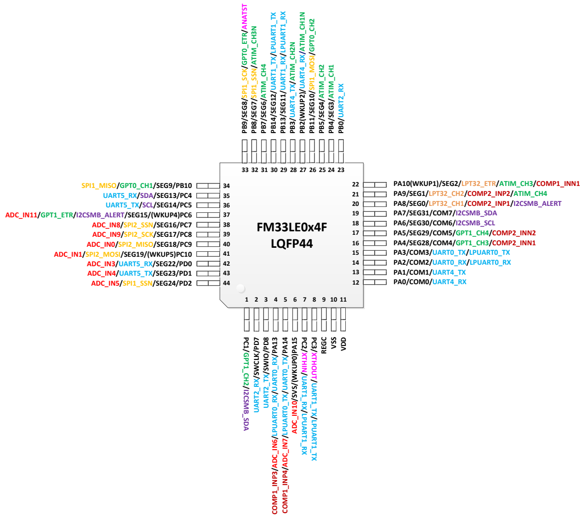
图 2-3FM33LE0x4F LQFP44 封装图
