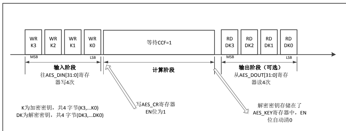
图 14-14 模式 2 示意图
