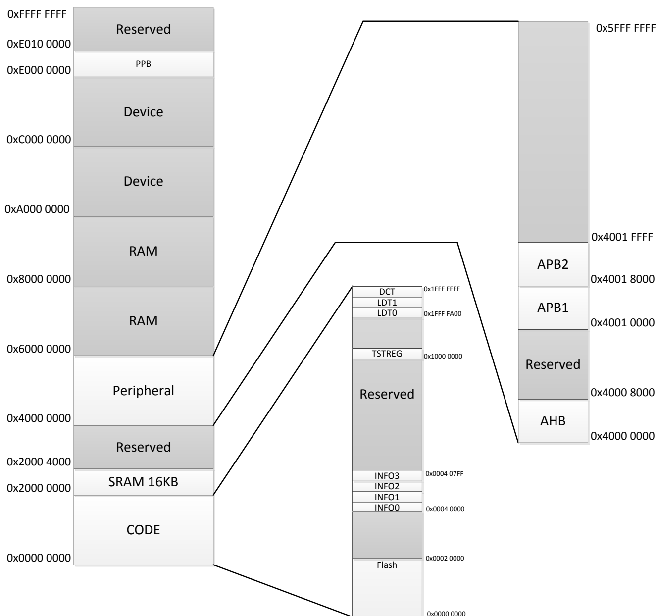
图 7-2FM33LE02x 总线地址
