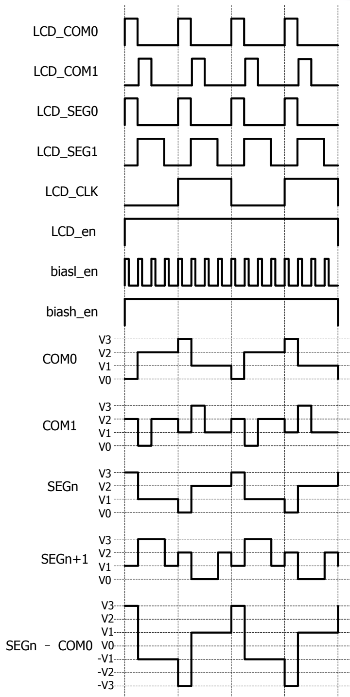
图 32-错误！未定义书签。 LCD 驱动波形(1/4 duty, 1/3 bias, type B)
