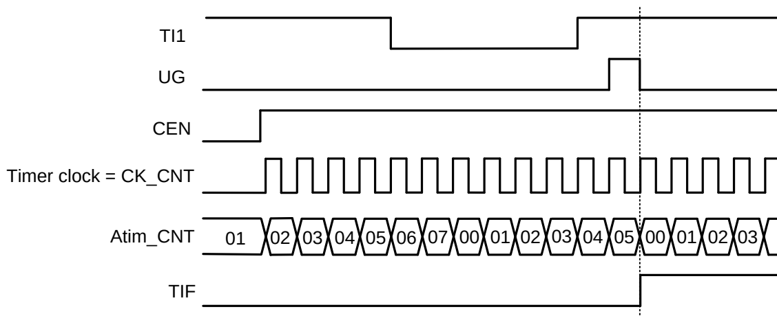
图27-40复位模式下的时序
