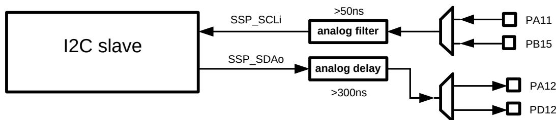
图 19-6 从机信号滤波
