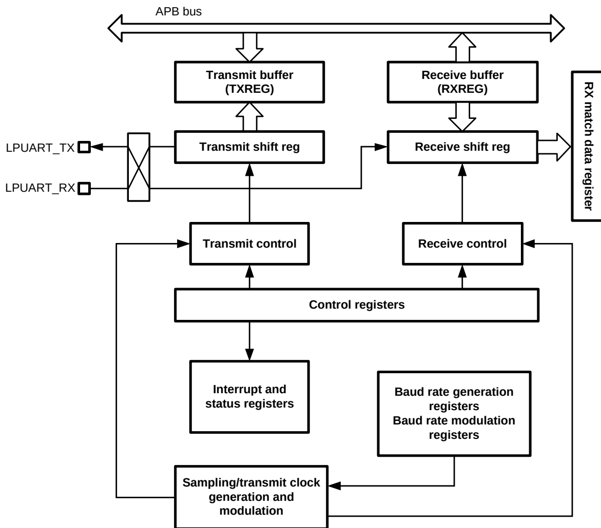
图 22-1LPUART 结构框图
