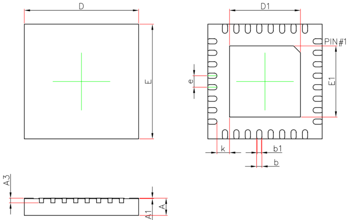
图 2-10 QFN32 封装尺寸图
