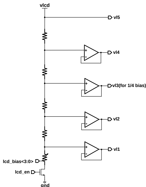
图 32-3LCD 片内电阻 buffer 型驱动电路
