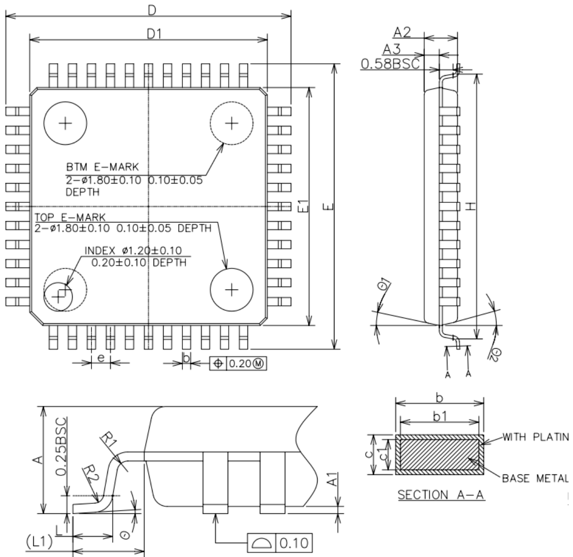
图 2-8 LQFP44 封装尺寸图
