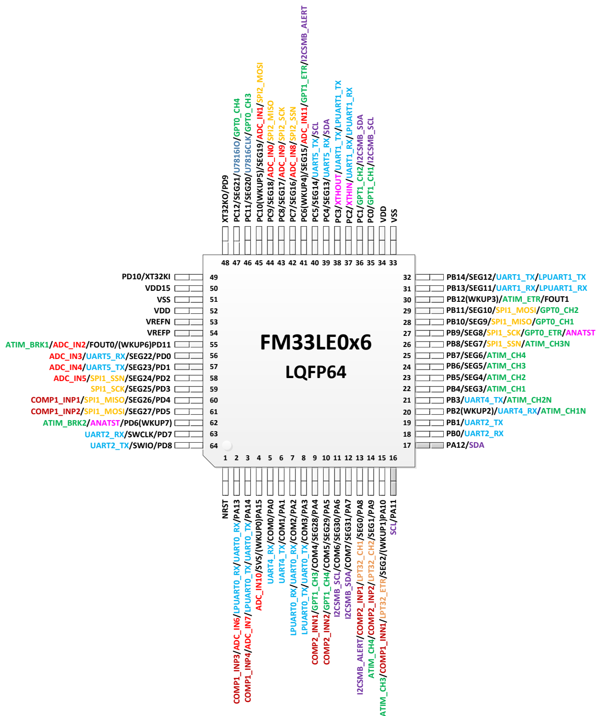
图 2-1FM33LE0x6 LQFP64 封装图
