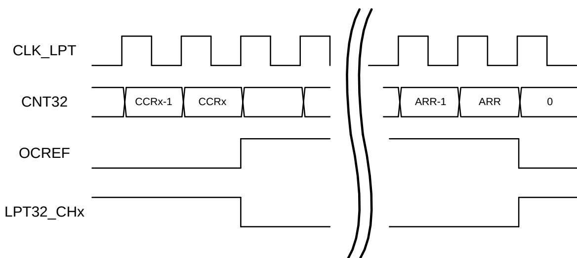
图 30-5 PWM 输出
