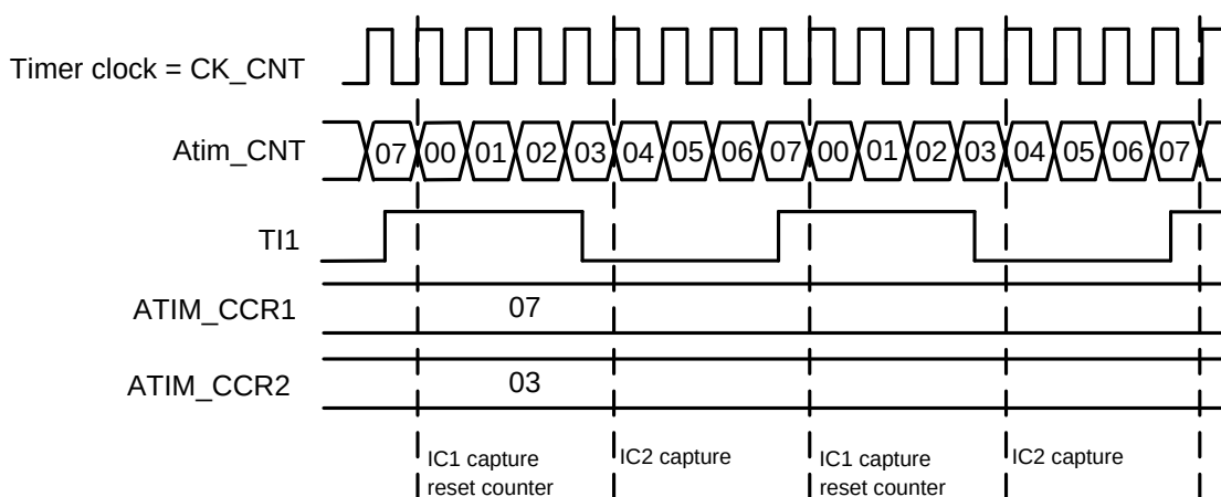
图27-28 PWM输入捕获模式时序
