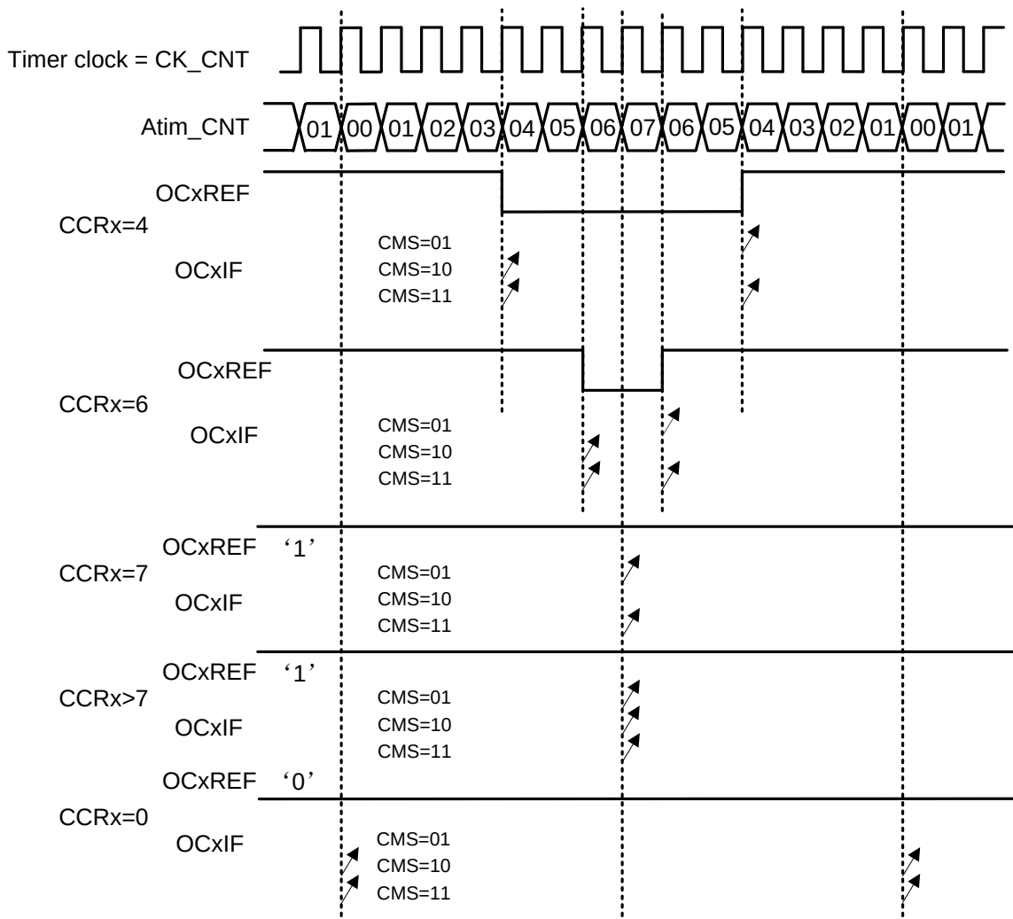
图27-31中央对齐的PWM波形(APR=7)
