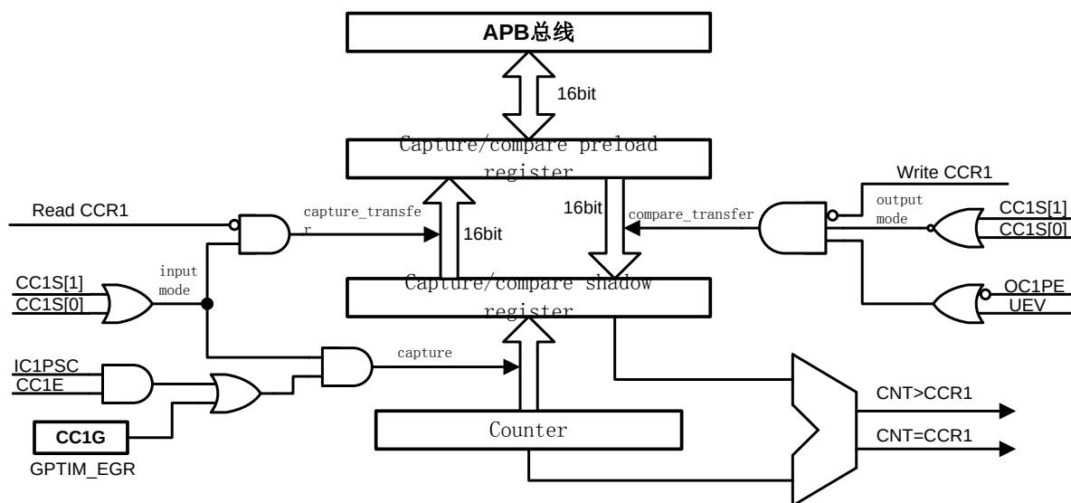
图28-24捕获/比较通道1的主电路
