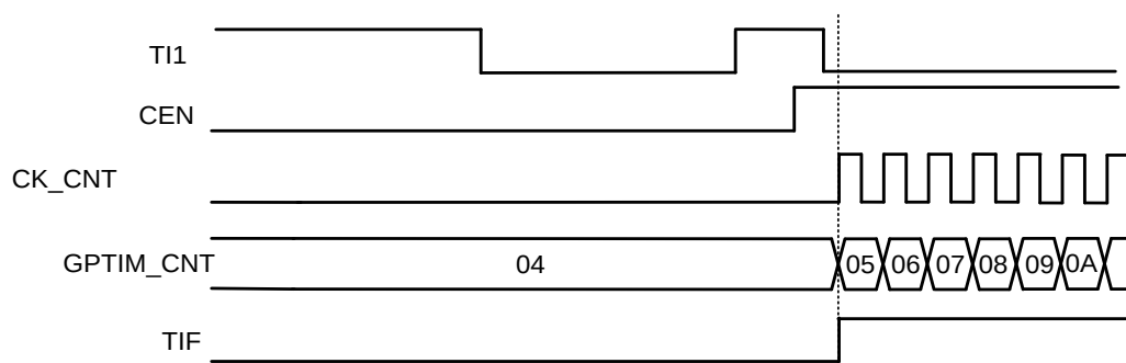
图28-35触发器模式下的时序
