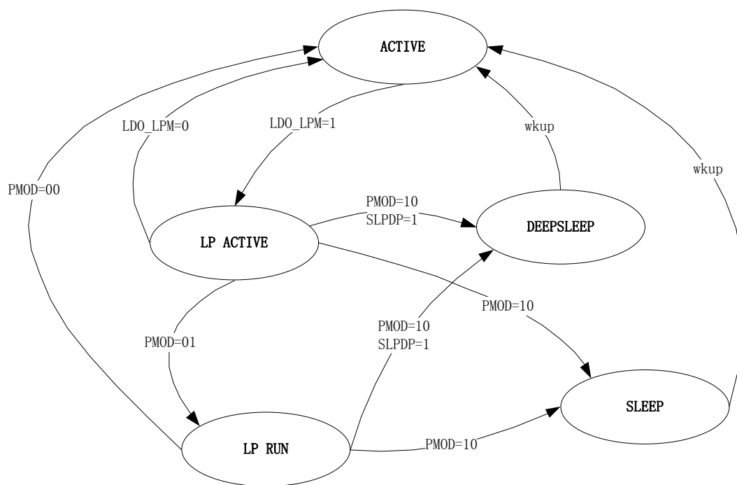
图 4-2 功耗模式转换
