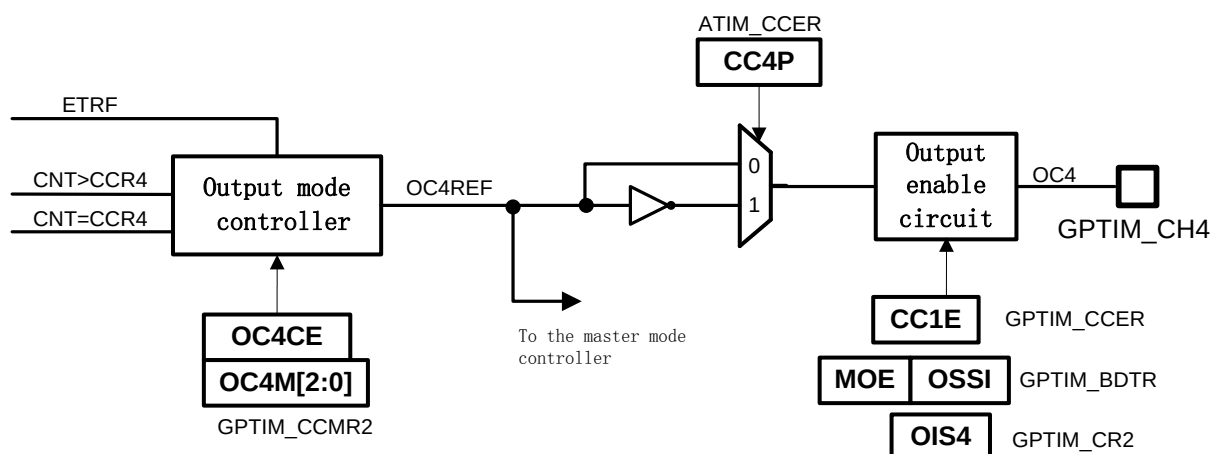
图28-25捕获/比较通道的输出部分
