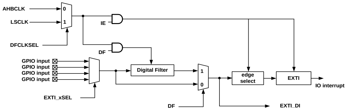
图 34-5 EXTI 信号输入示意图
