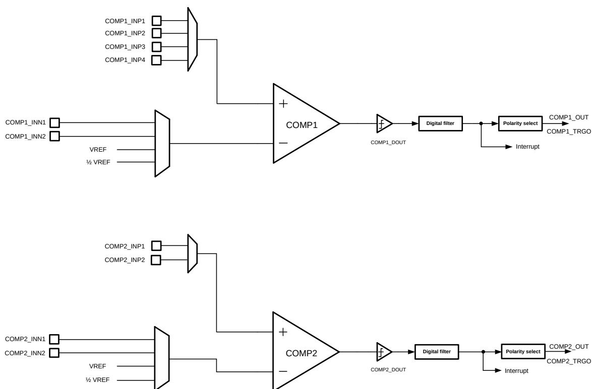
图 16-1 比较器电路框图
