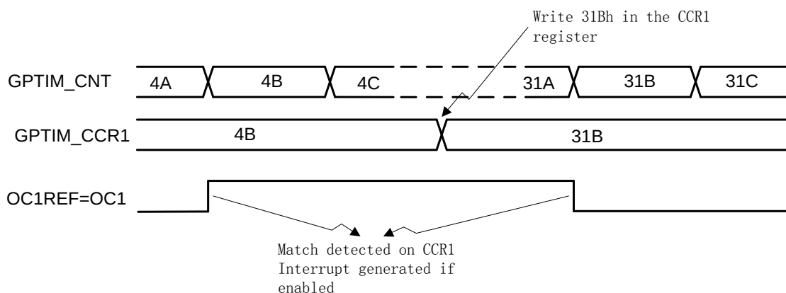
图28-27输出比较模式，翻转OC1
