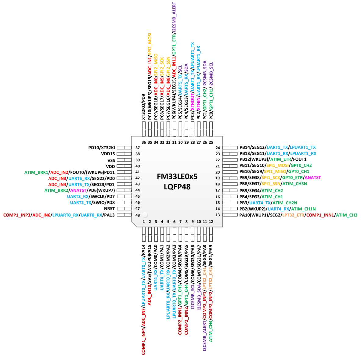
图 2-2FM33LE0x5 LQFP48 封装图
