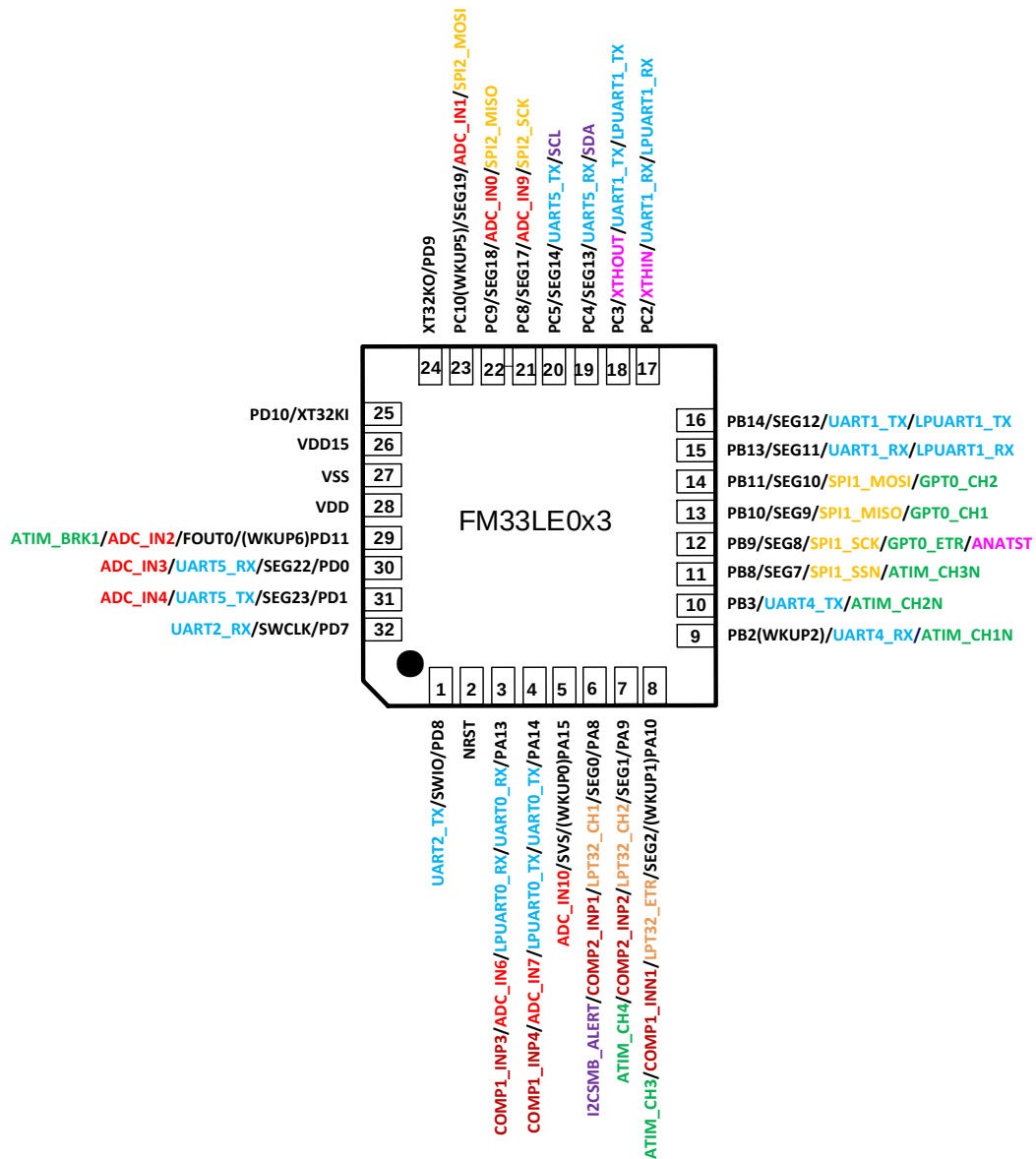
图 2-5FM33LE0x3QFN32 封装图
