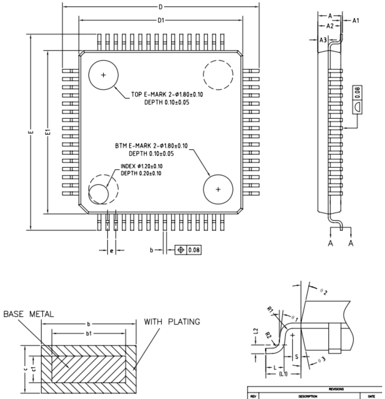
图 2-6 LQFP64 封装尺寸图
