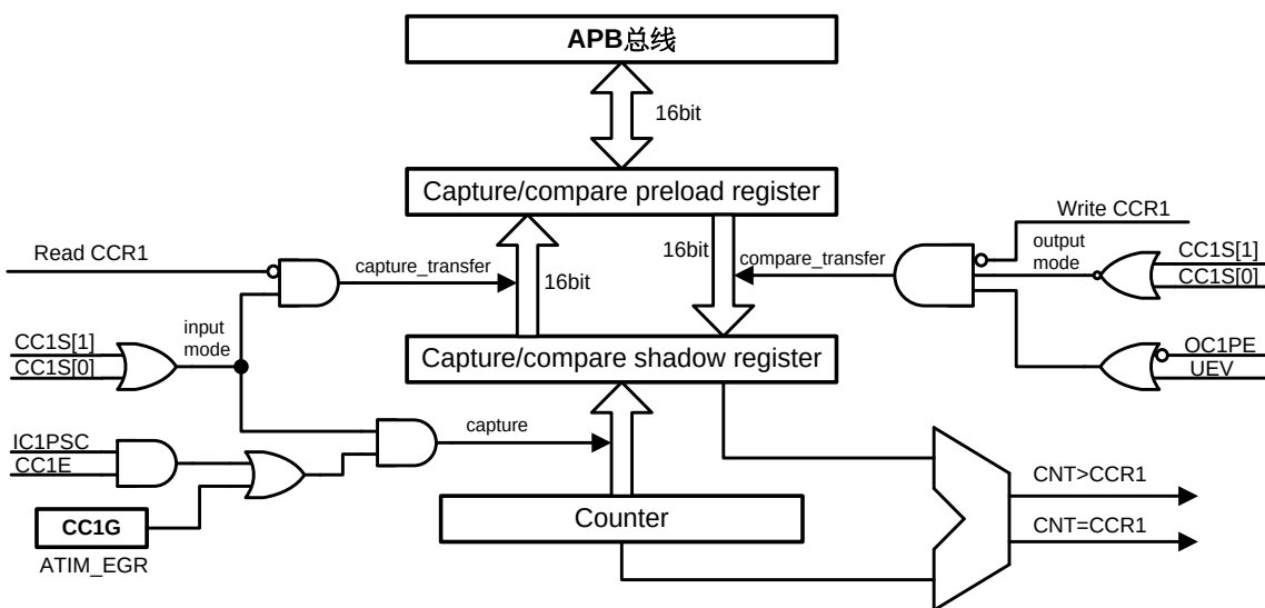
图27-25捕获/比较通道1的主电路
