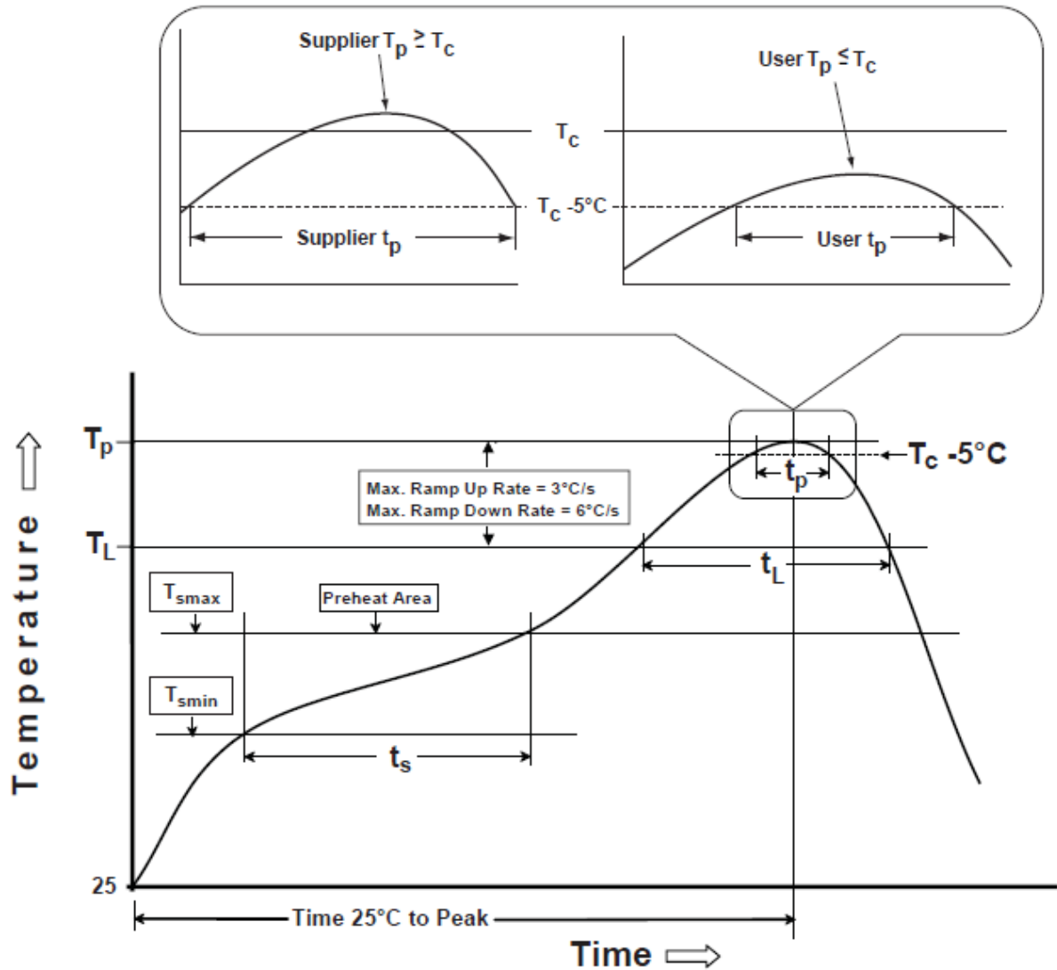
图 2-11JEDEC 标准的耐热回流温度曲线
