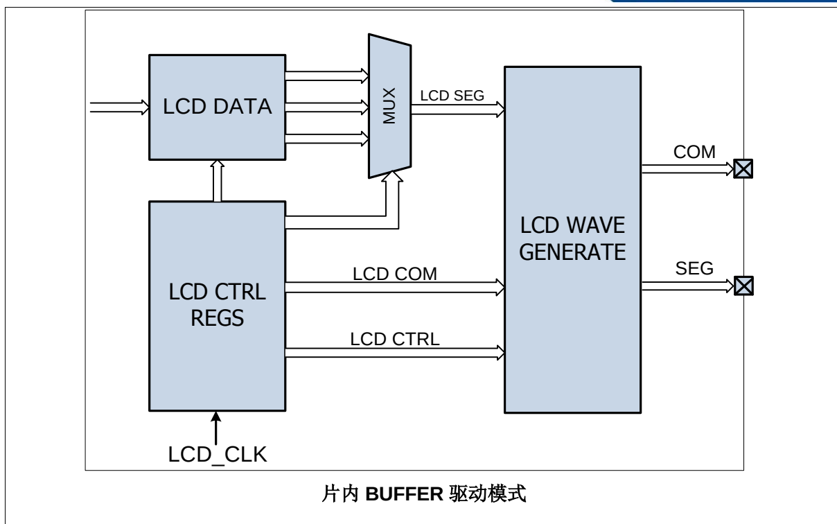
图 32-1 LCD 显示控制模块结构框图
