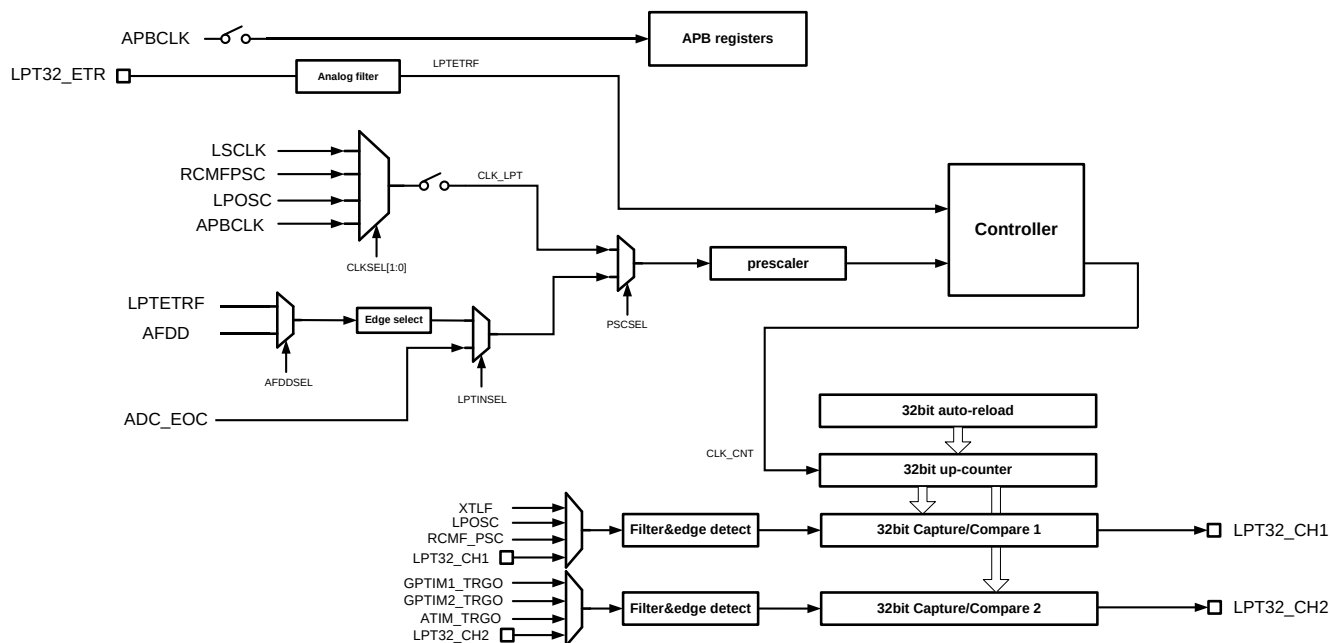
图 30-1 LPTIM32 结构框图
