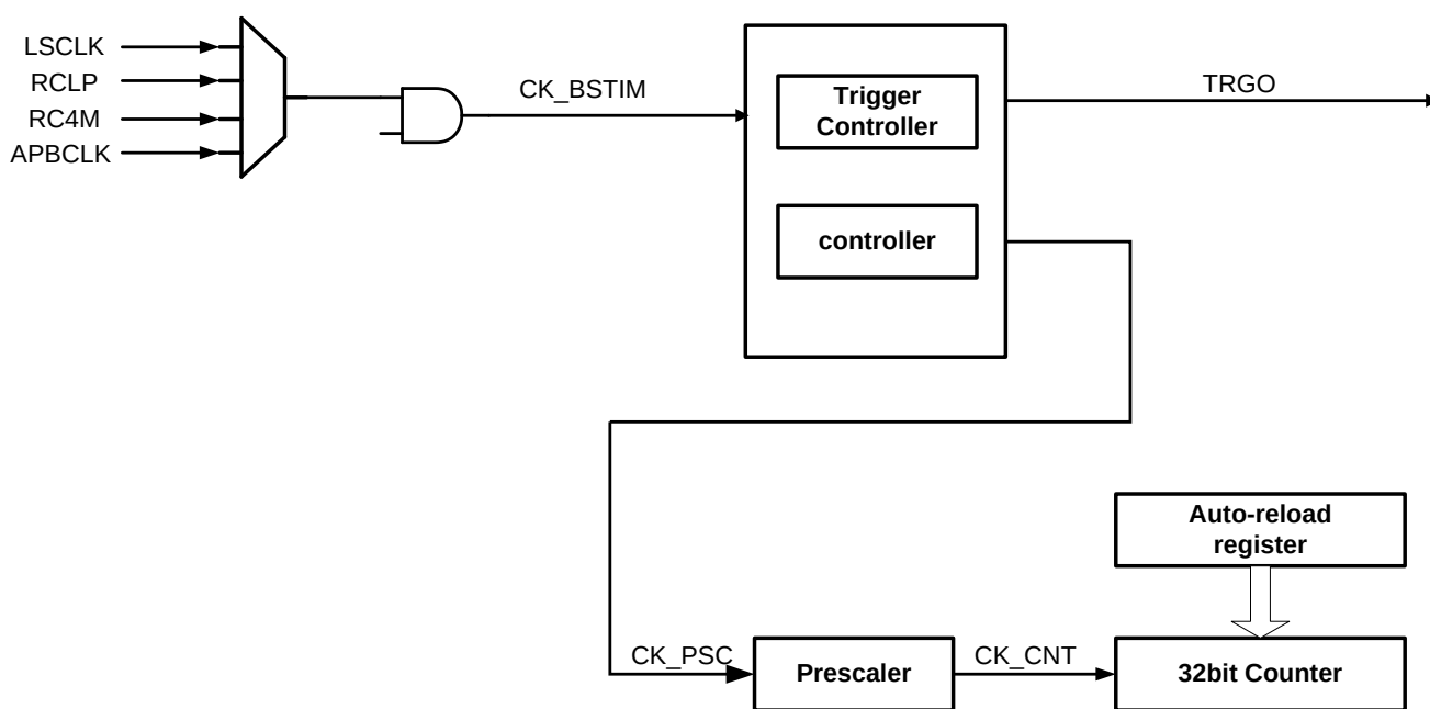
图29-1BSTIM32结构框图
