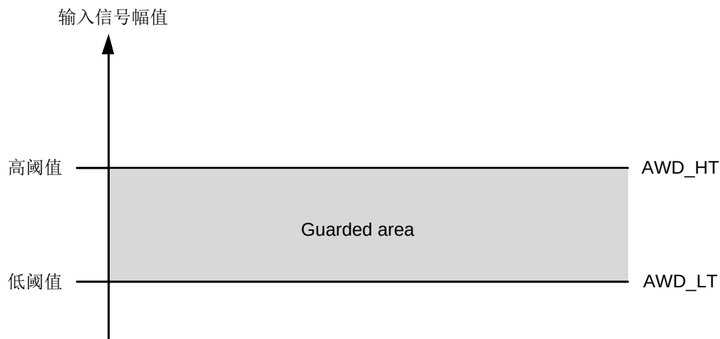
图 33-13 ADC 模拟看门狗阈值示意图
