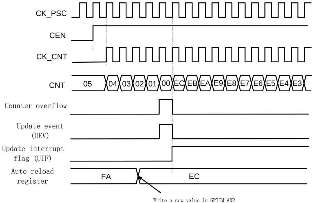
图 28-11 向下计数，不使用重复计数时的更新事件
