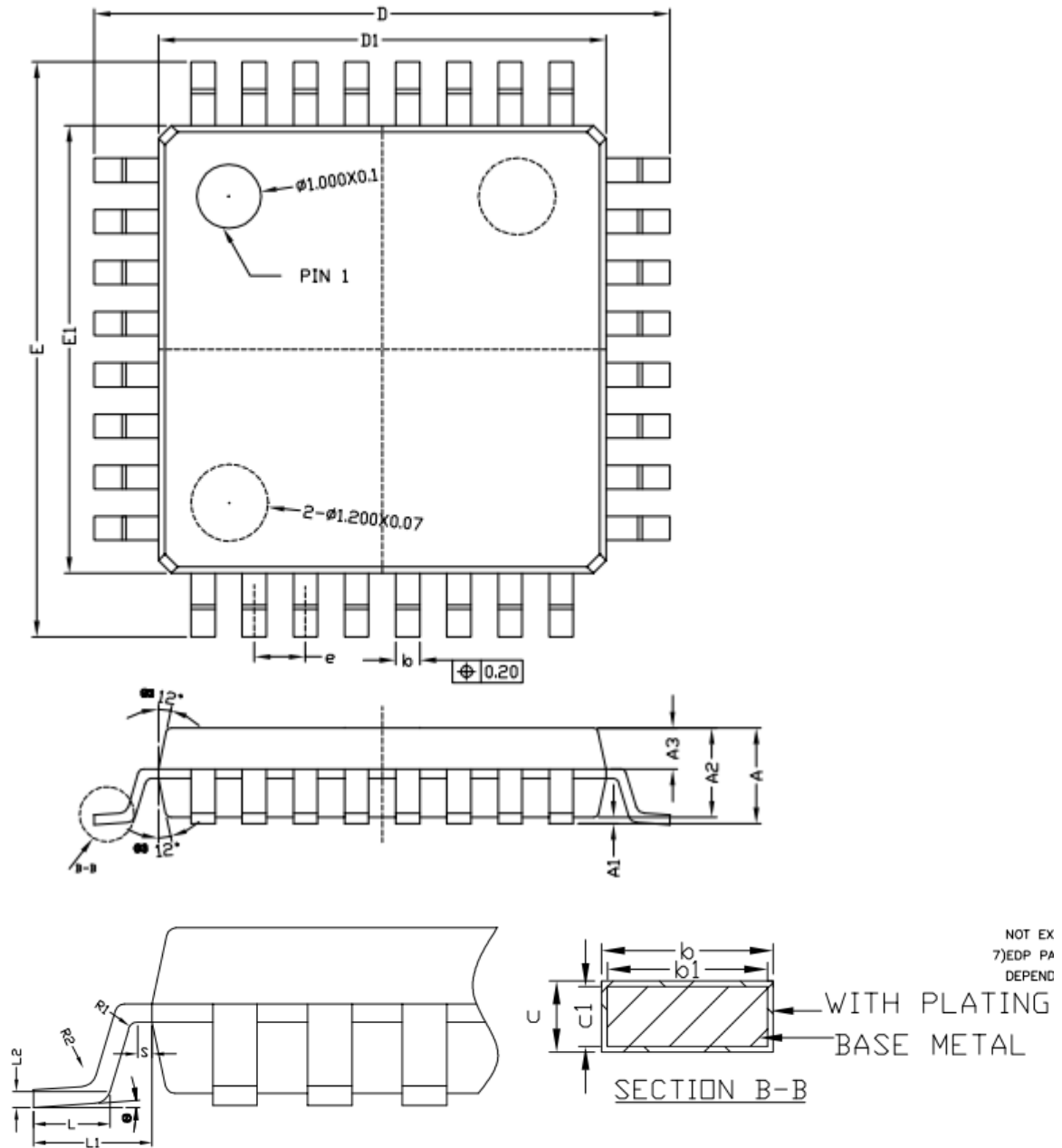
图 2-9LQFP32 封装尺寸图
