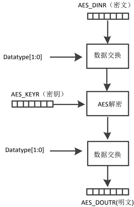
图 14-2 ECB 模式解密流程
