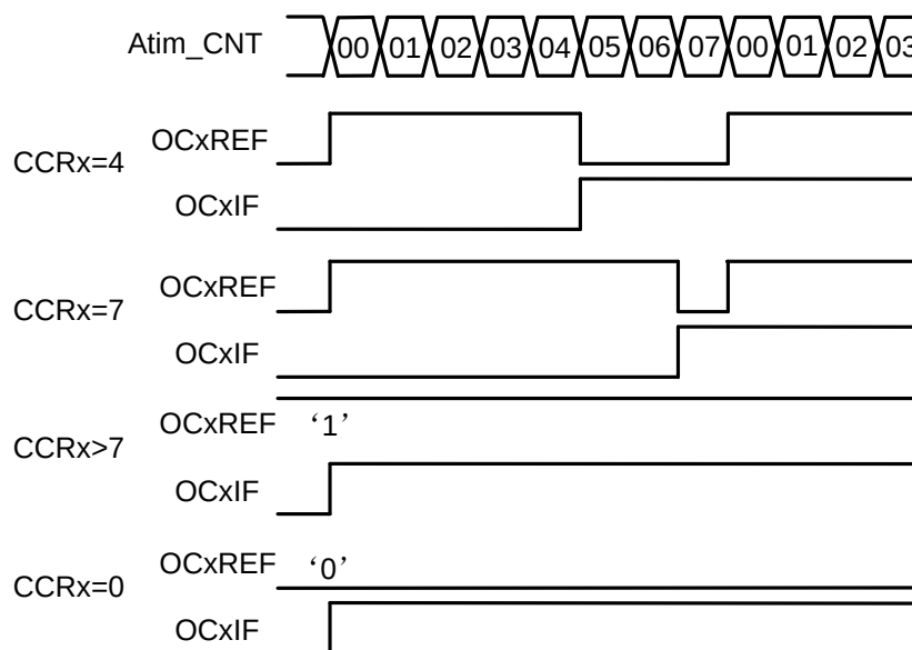
图27-30边沿对齐的PWM波形(ARR=7)
