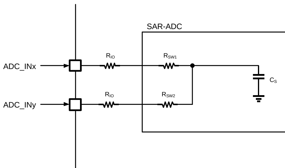
图 33-5 ADC 输入通道示意图
