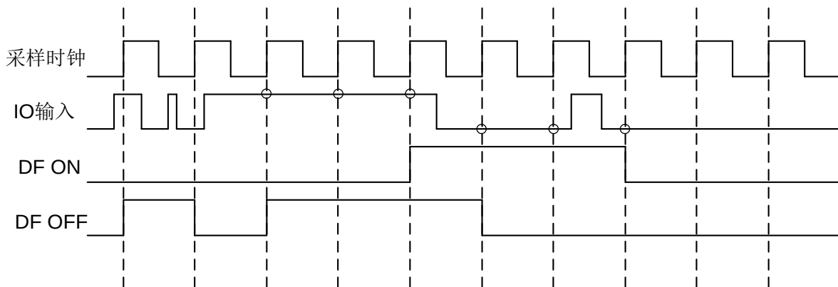
图 34-4 引脚输入数字滤波
