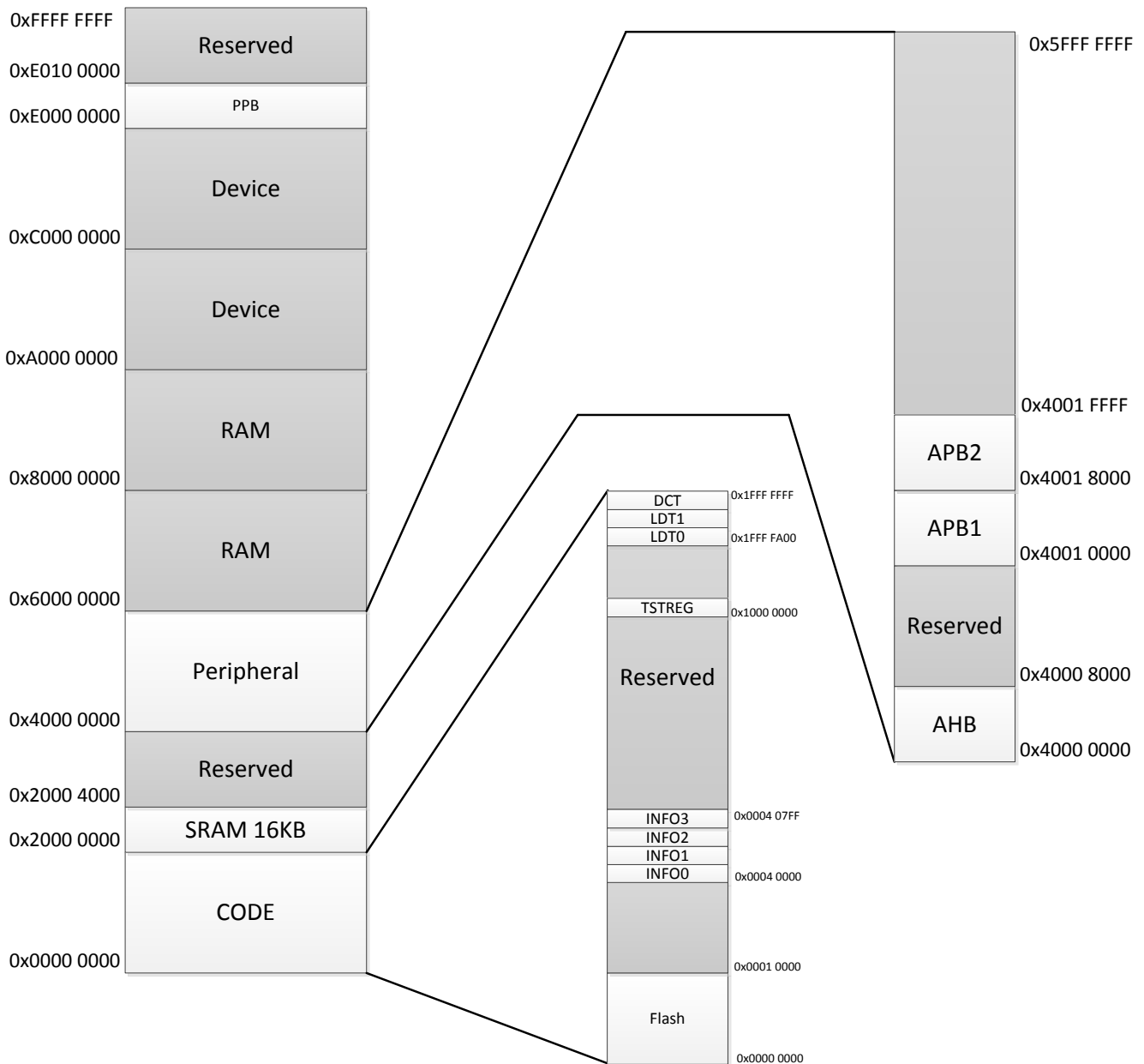
图 7-3FM33LE01x 总线地址
