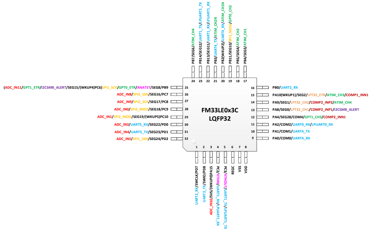
图 2-4FM33LE0x3C LQFP32 封装图
