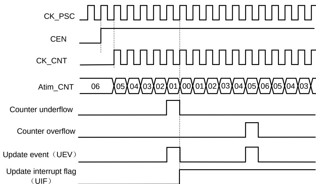
图 28-12 中心对齐计数器时序图，GPTIM_PCS=0，GPTIM_ARR=0x6
