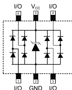
SOT-363
