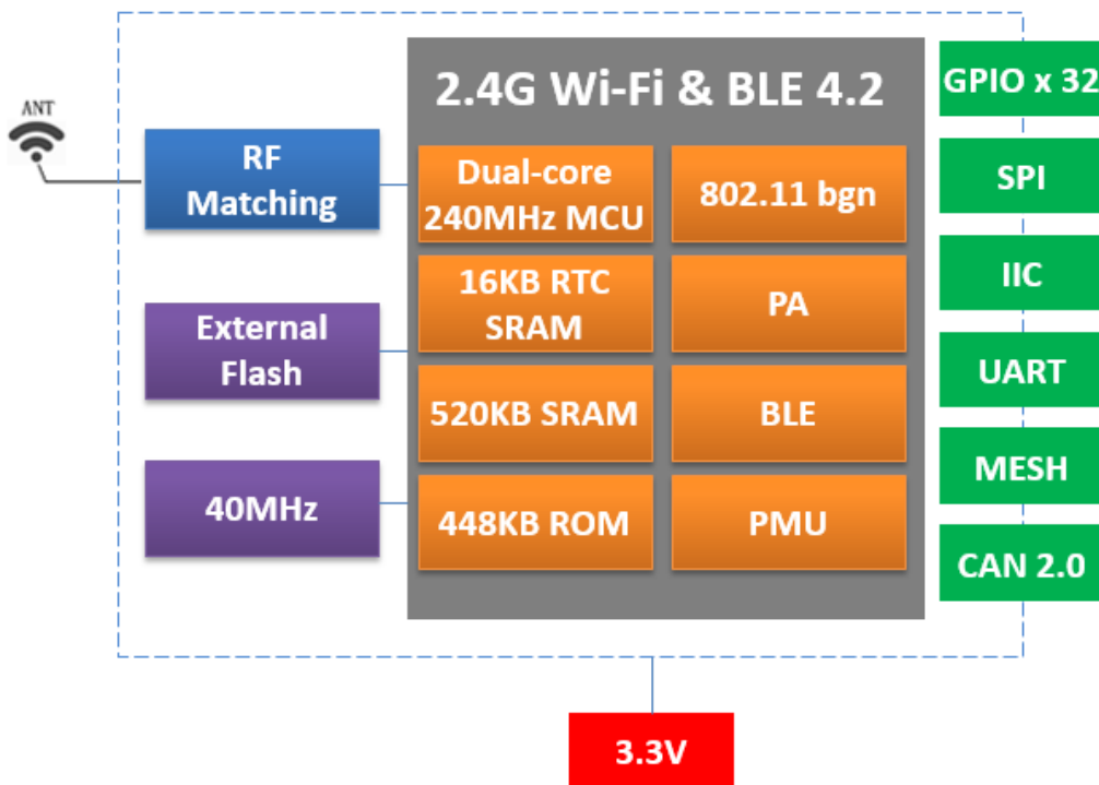
Fig.1.1 ESP32-32E Module Structure
