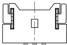
结构外形(锁扣窗口)
