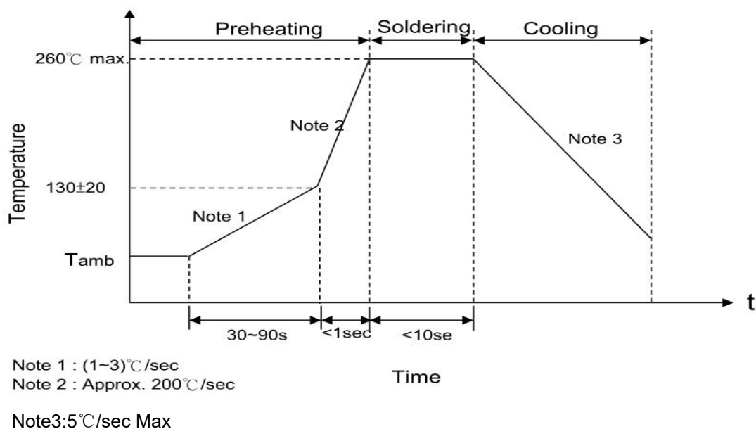
(图 2: 波峰焊曲线图)
