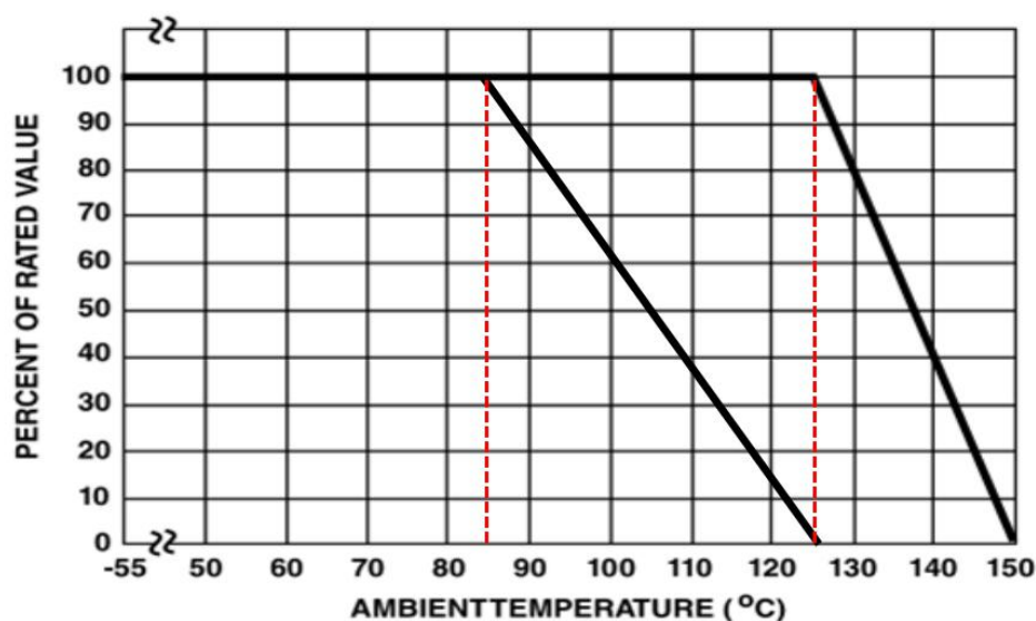
(图 1: 电流、能量、功率递减曲线)
