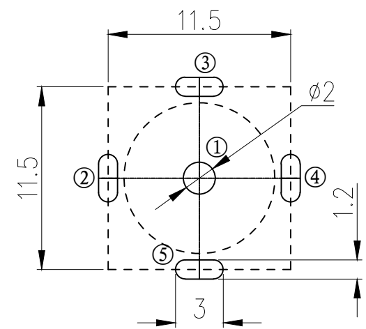
PCB LAYOUT (TOP VIEW) P. C. B开孔示意图
