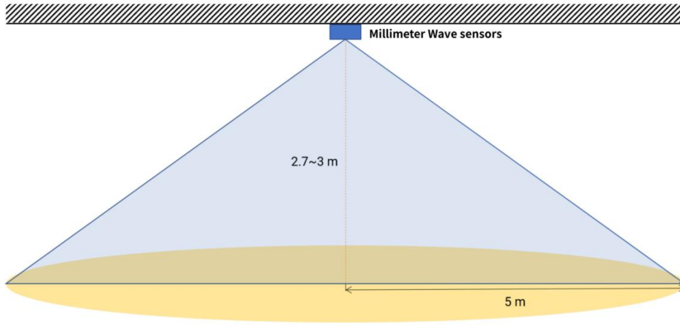
图 5-2 E54-05LD06系列挂顶安装检测范围示意图
